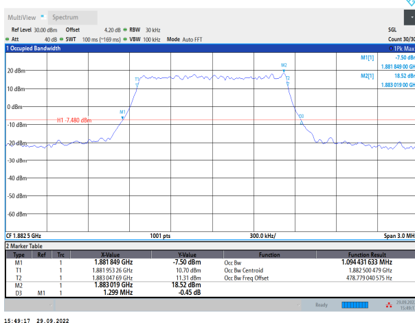
Band25-1.4MHz-QPSK-26365-6RB#0
