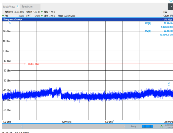
Band25-20MHz-QPSK-26140-1RB#0-Range4:1000~20000MHz
