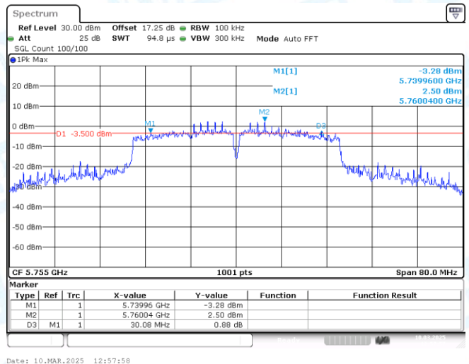
11N40MIMO-Ant1-5755-PASS
