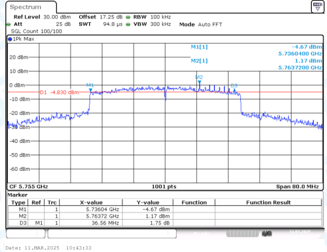
11AX40MIMO-Ant1-5755-PASS
