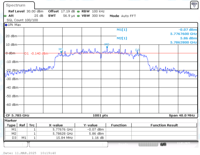
11AX20MIMO-Ant1-5785-PASS
