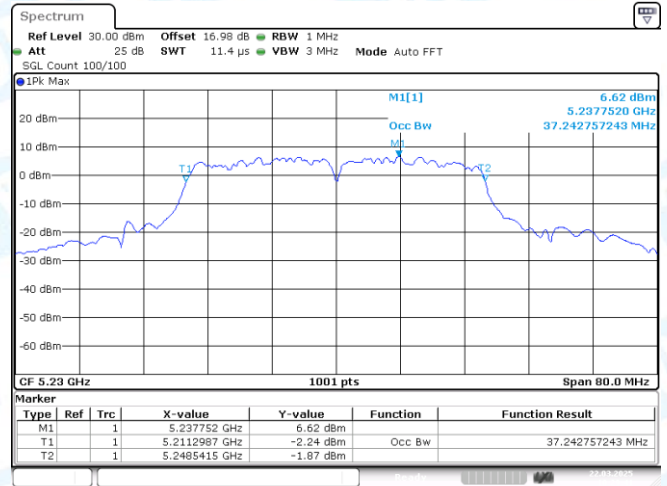
11AX40MIMO-Ant1-5230
