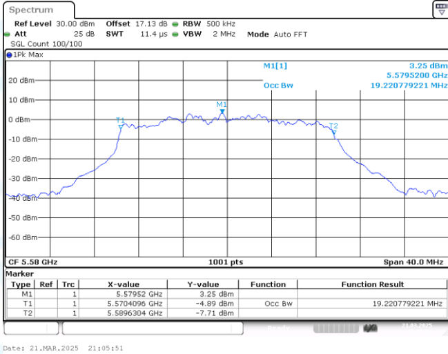
11AX20MIMO-Ant2-5580
