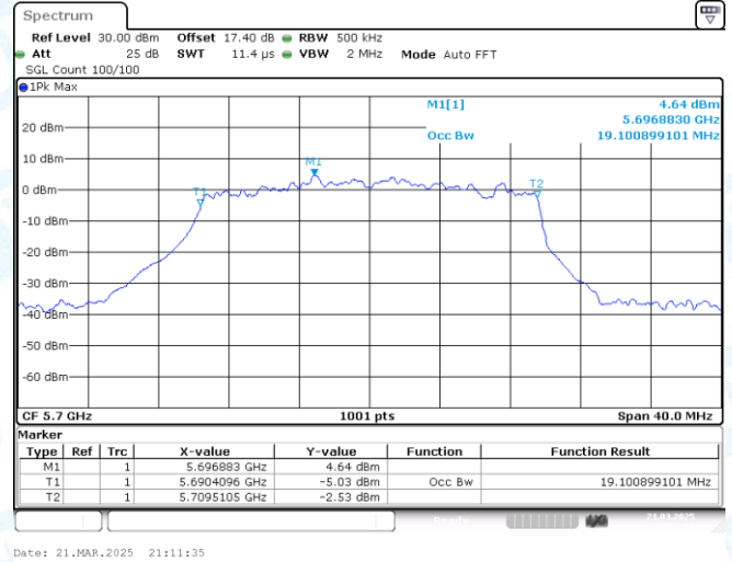
11AX20MIMO-Ant1-5700
