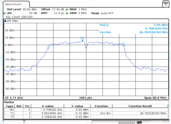
11AX40MIMO-Ant1-5710
