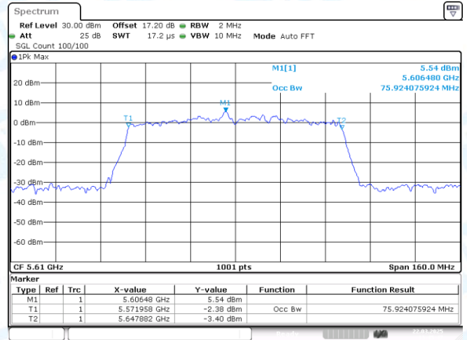
11AX80MIMO-Ant1-5610
