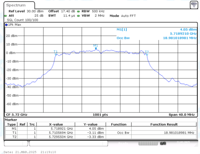
11AX20MIMO-Ant1-5720
