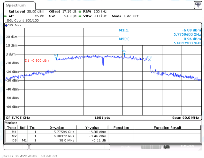
11AX40MIMO-Ant1-5795-PASS
