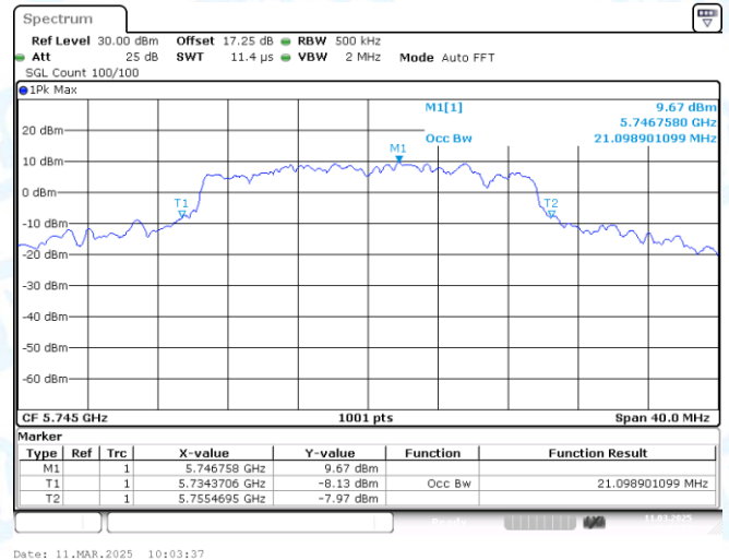
11AX20MIMO-Ant1-5745
