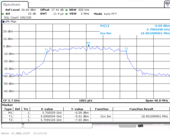
11AX20MIMO-Ant2-5700
