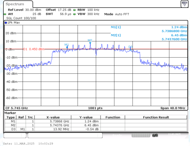
11AX20MIMO-Ant1-5745-PASS
