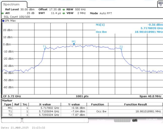
11AX20MIMO-Ant2-5720
