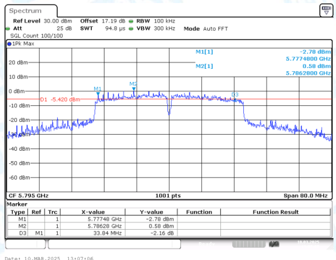
11N40MIMO-Ant1-5795-PASS
