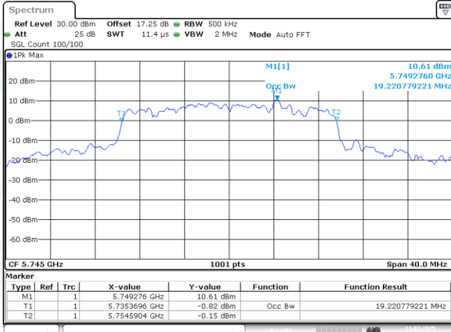
11AX20MIMO-Ant2-5745
