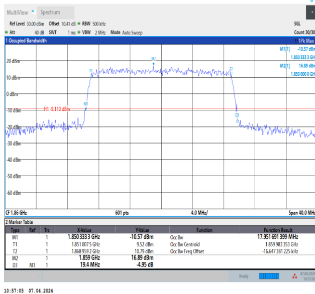
Band2-20MHz-16QAM-18700-100RB#0-PASS
