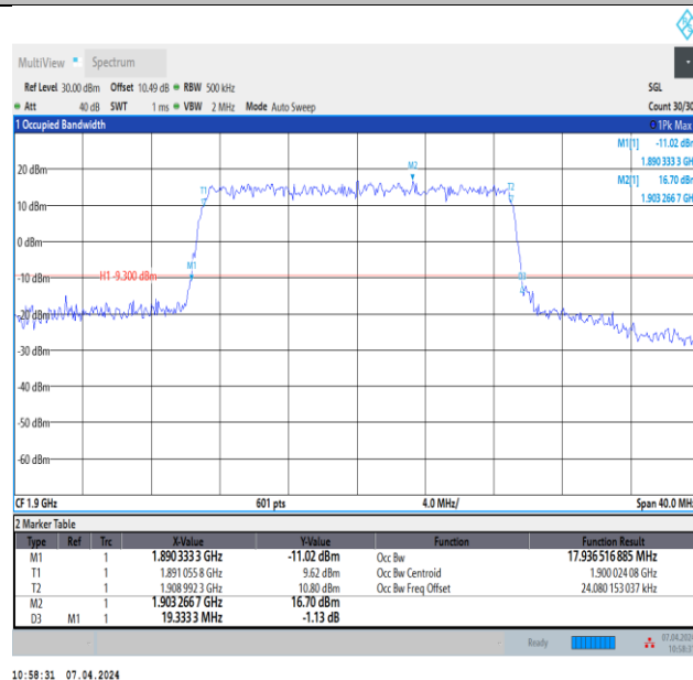
Band2-20MHz-QPSK-19100-100RB#0-PASS
