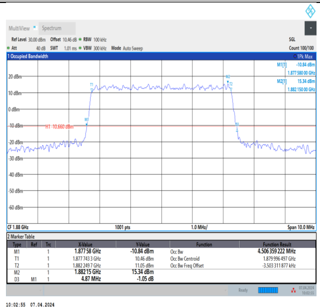
Band2-5MHz-QPSK-18900-25RB#0-PASS
