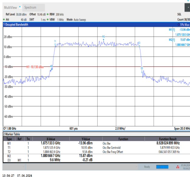
Band2-10MHz-QPSK-18900-50RB#0-PASS
