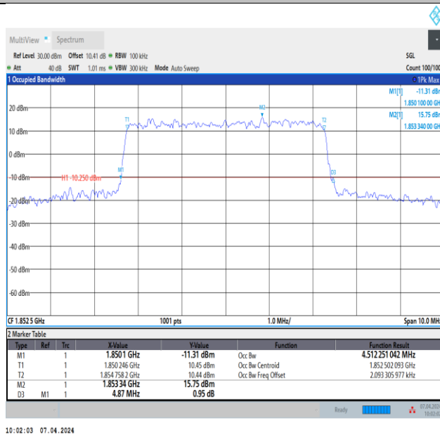
Band2-5MHz-QPSK-18625-25RB#0-PASS
