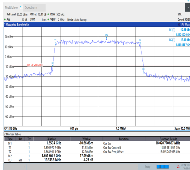
Band2-20MHz-QPSK-18700-100RB#0-PASS
