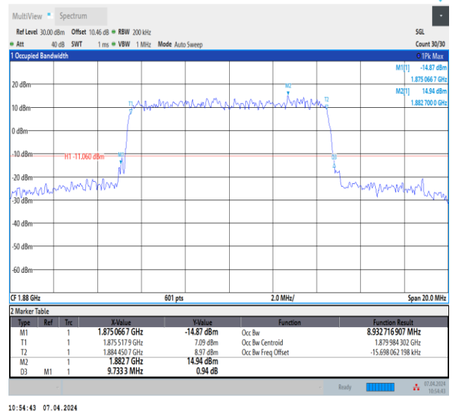
Band2-10MHz-16QAM-18900-50RB#0-PASS
