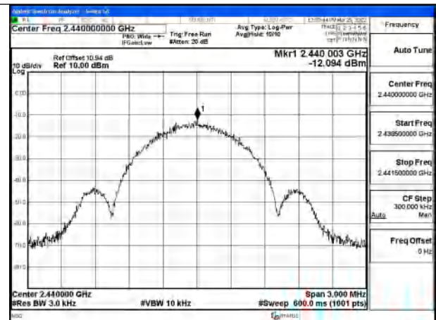
Test Mode:GFSK (LE 1Mbps) MHz
