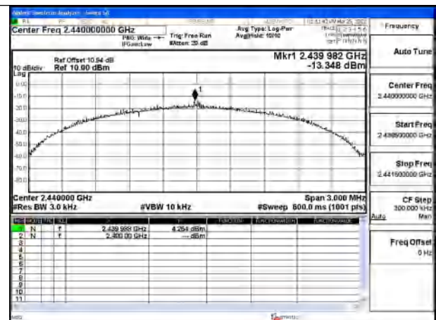
Test Mode:GFSK (LE 2Mbps) MHz
