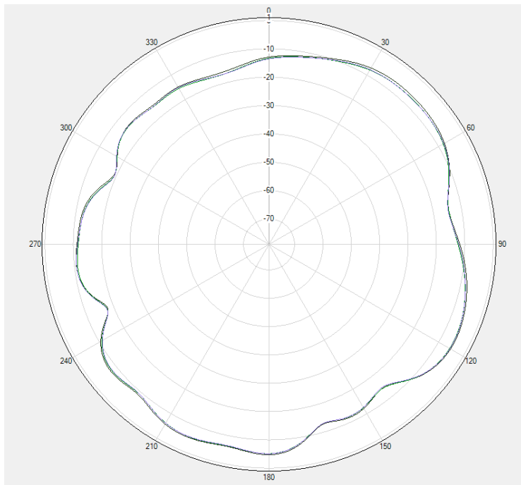
GPS \Phi=0^\circ
