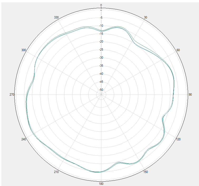
GPS \Phi=90^\circ
