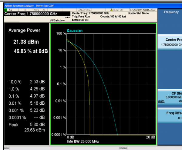
Band4-10MHz-QPSK-20350-1RB#0-PASS
