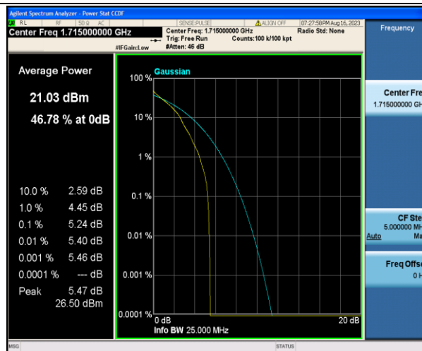
Band4-10MHz-QPSK-20000-1RB#0-PASS
