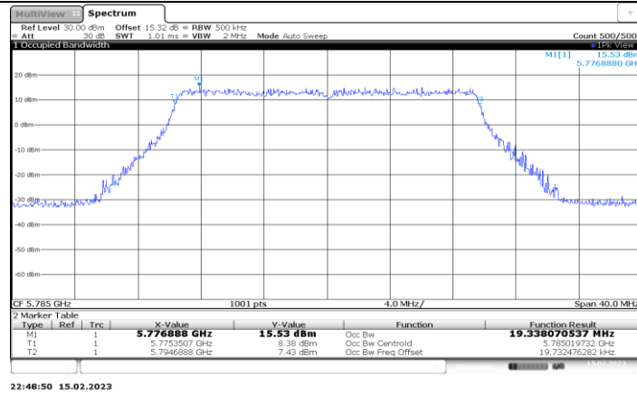
11BE20MIMO_Ant3_5785
