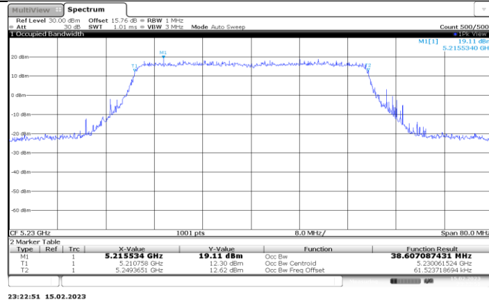
11BE40MIMO_Ant2_5230
