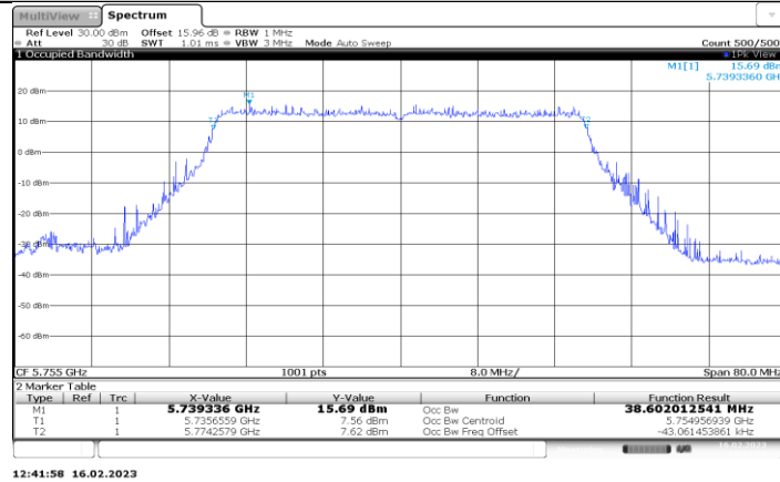
11BE40MIMO_Ant2_5755
