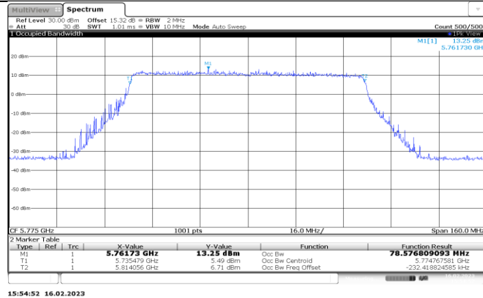
11BE80MIMO_Ant3_5775
