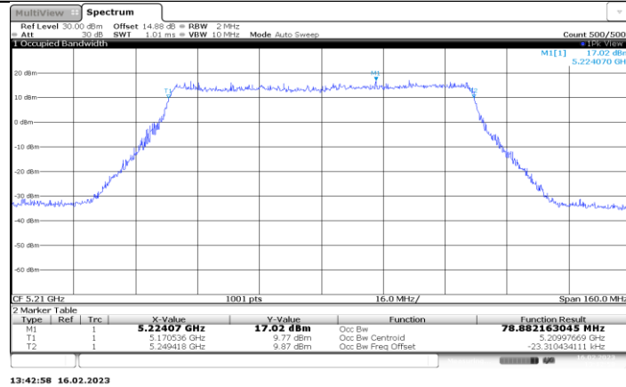
11BE80MIMO_Ant3_5210
