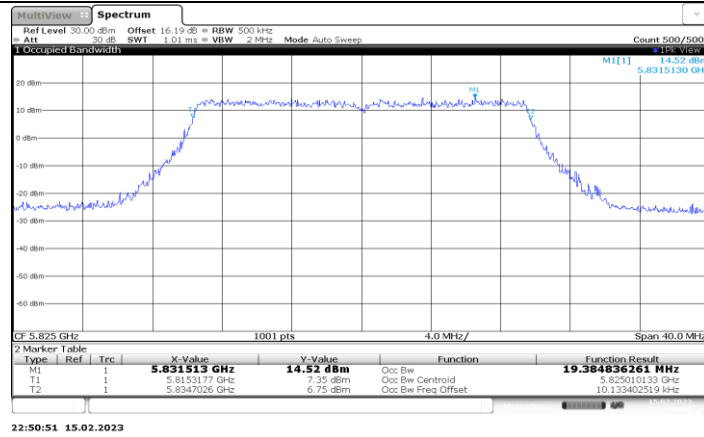
11BE20MIMO_Ant2_5825
