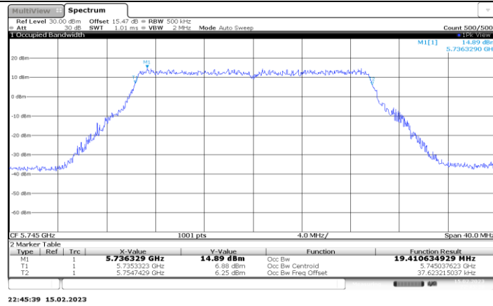
11BE20MIMO_Ant4_5745
