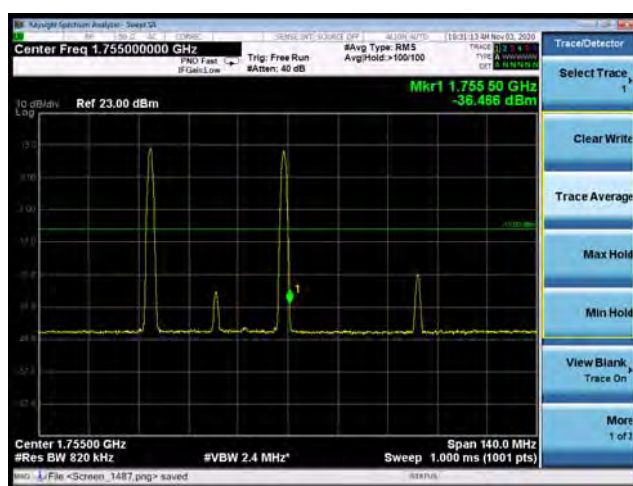
CA-4C-12A 64QAM 20MHz+20MHz+20MHz CH-High, 100%RB
