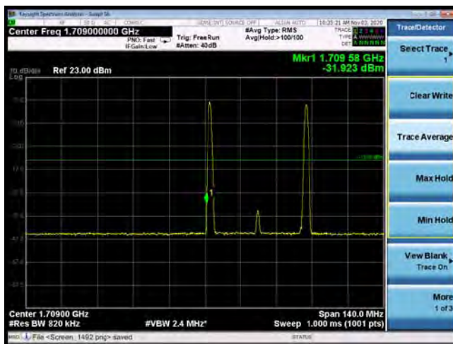
CA-4C-12A 16QAM 20MHz+20MHz+20MHz CH-Low, 1 RB
