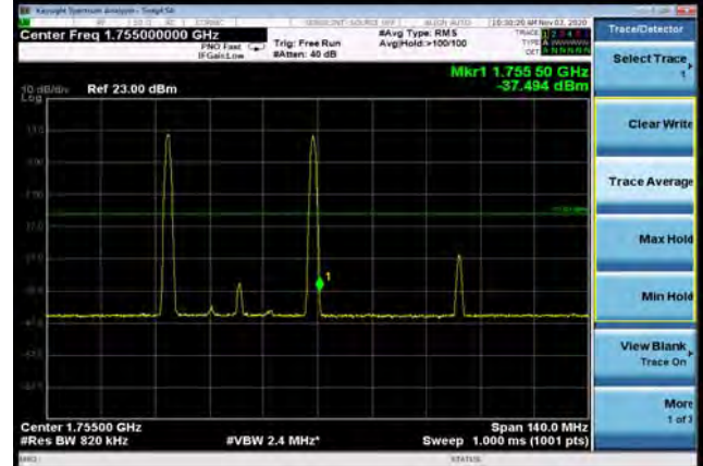
CA-4C-12A QPSK 20MHz+20MHz+20MHz CH-High, 100%RB
