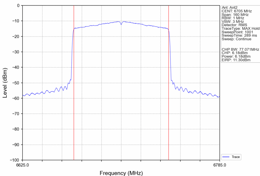
802.11ax(HEW80)_MCH_6705MHz_RU996_Left_Ant2_NTNV
