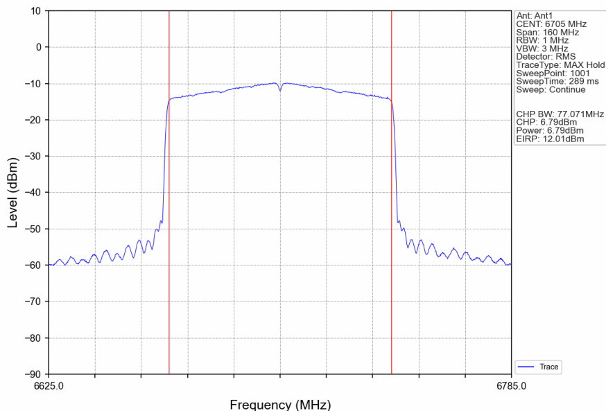
802.11ax(HEW80)_MCH_6705MHz_RU996_Left_Ant1_NTNV
