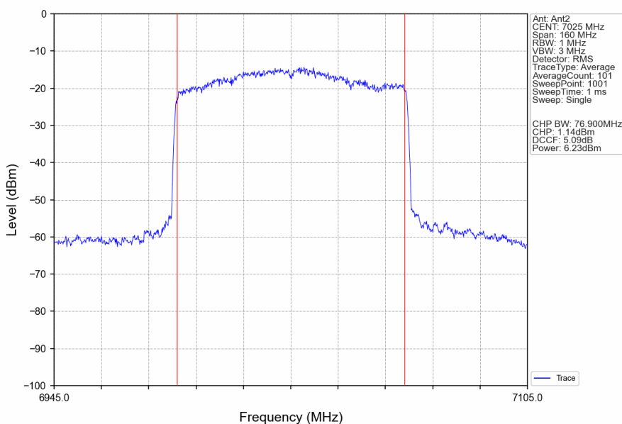
802.11ax(HEW80)_HCH_7025MHz_RU996_Left_Ant2_NTNV
