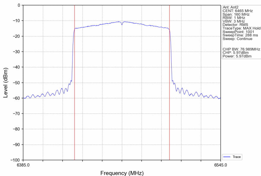
802.11ax(HEW80)_LCH_6465MHz_RU996_Left_Ant2_NTNV
