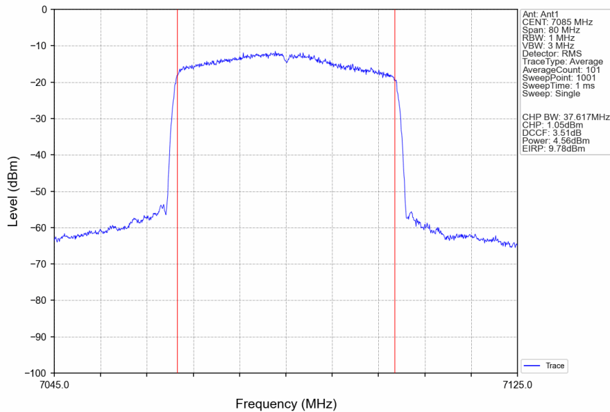
802.11ax(HEW40)_HCH_7085MHz_RU484_Left_Ant1_NTNV
