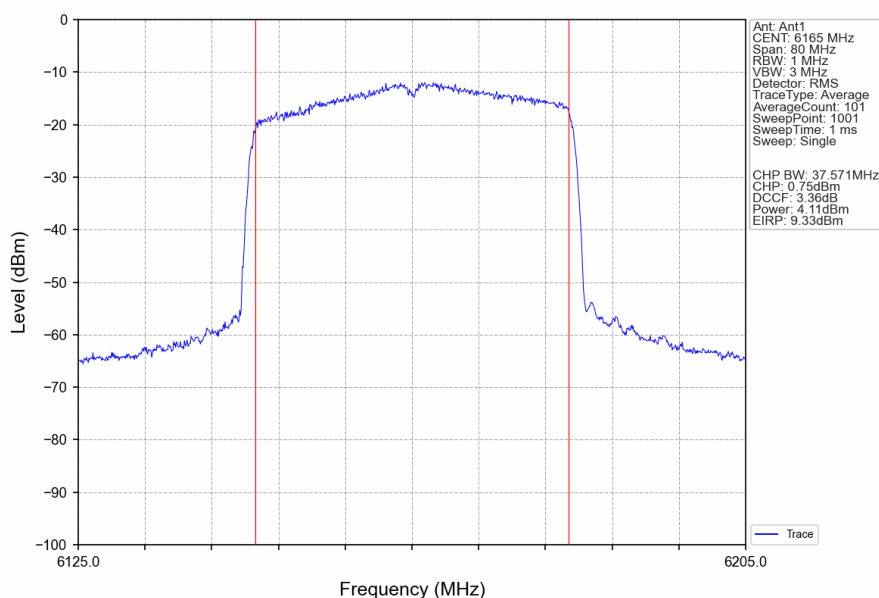
802.11ax(HEW40)_MCH_6165MHz_RU484_Left_Ant1_NTNV
