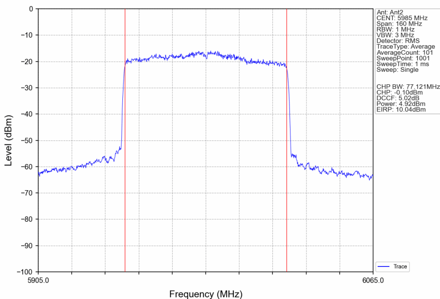
802.11ax(HEW80)_LCH_5985MHz_RU996_Left_Ant2_NTNV
