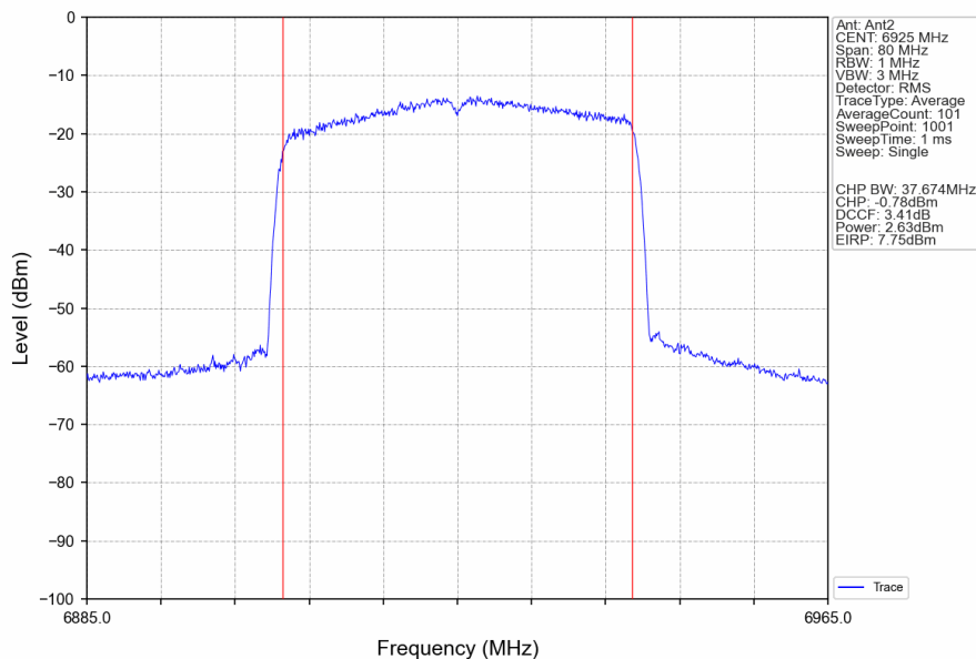
802.11ax(HEW40)_LCH_6925MHz_RU484_Left_Ant2_NTNV
