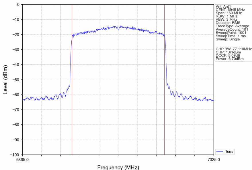
802.11ax(HEW80)_LCH_6945MHz_RU996_Left_Ant1_NTNV
