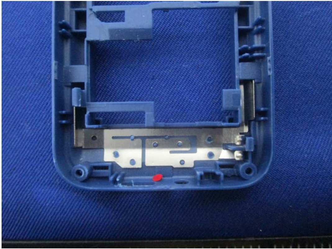
GSM Antenna
