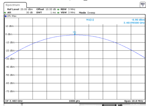
\pi/4 -DQPSK_Low
