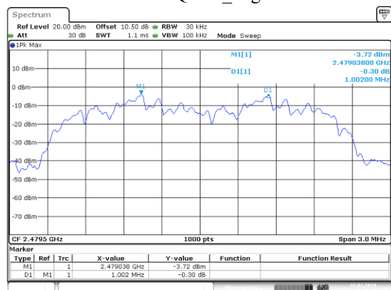
\pi/4 -DQPSK_High
