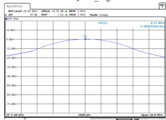
\pi/4 -DQPSK_High
