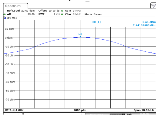
\pi/4 -DQPSK_Middle
