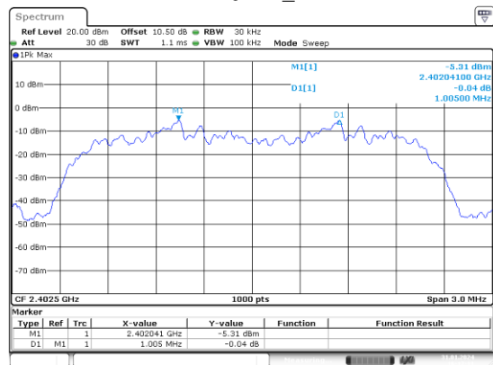
\pi/4 -DQPSK_Low
