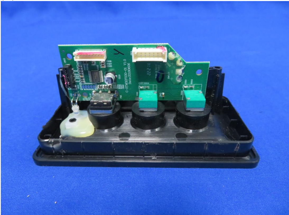
(14) EUT Photo
