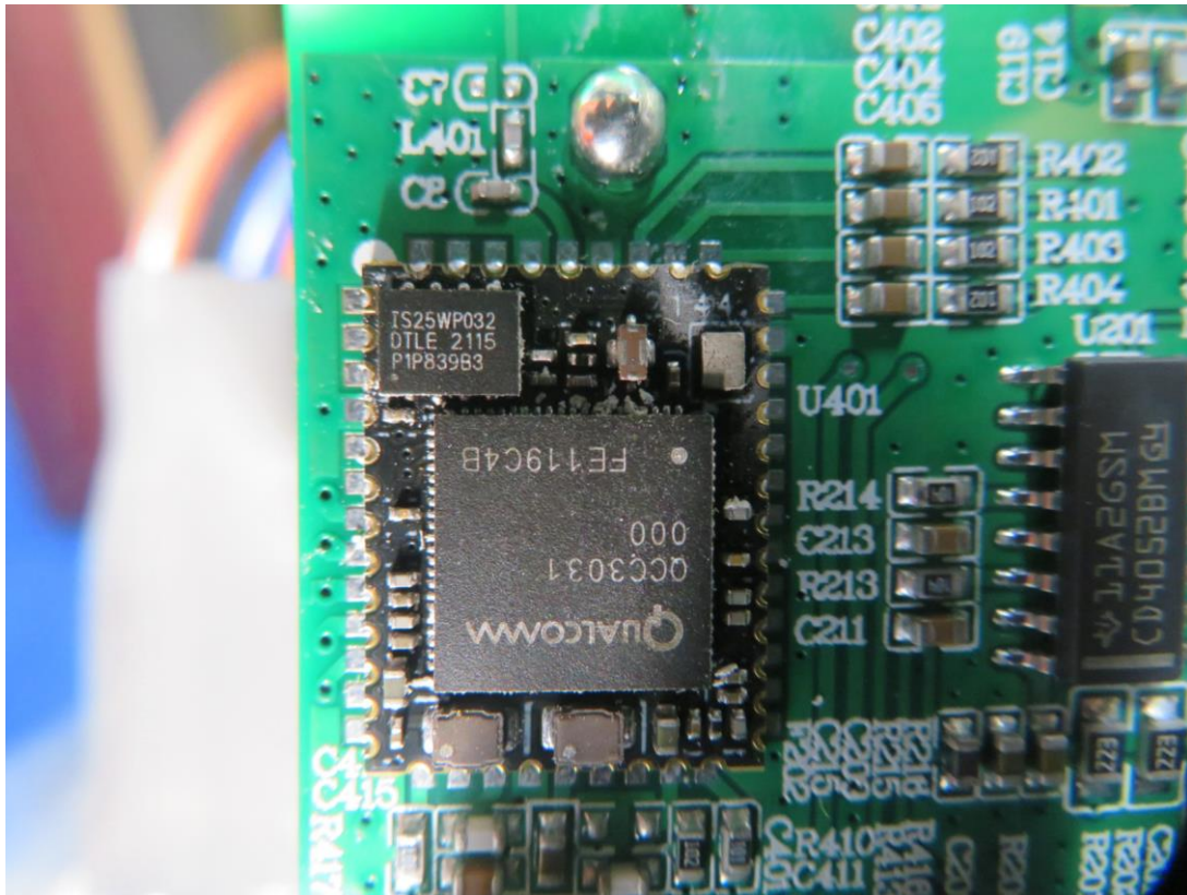
(4) EUT Photo
