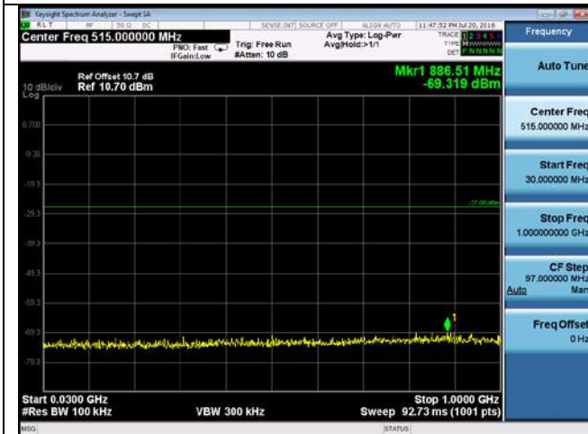
CUE-802.11n-20-5700M -chain 1(30MHz-1GHz)
