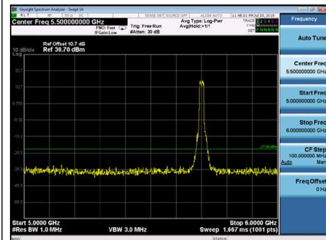
CUE-802.11n-20-5700M -chain 1(5GHz-6GHz)
