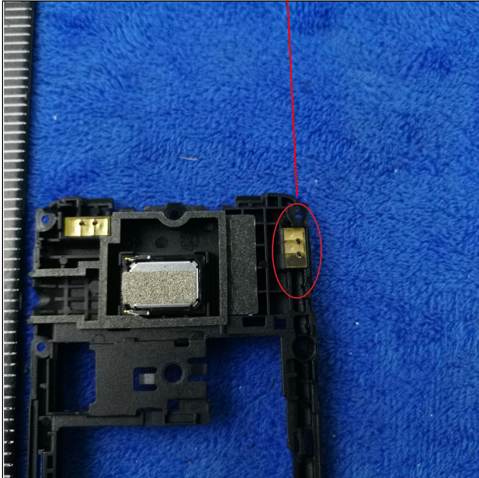
BT/WIFI/GPS Antenna
