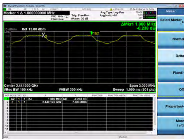
GFSK
