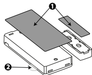
Figura 2: Instalação rápida 1: Fita adesiva dupla face 2: Aba Registro
