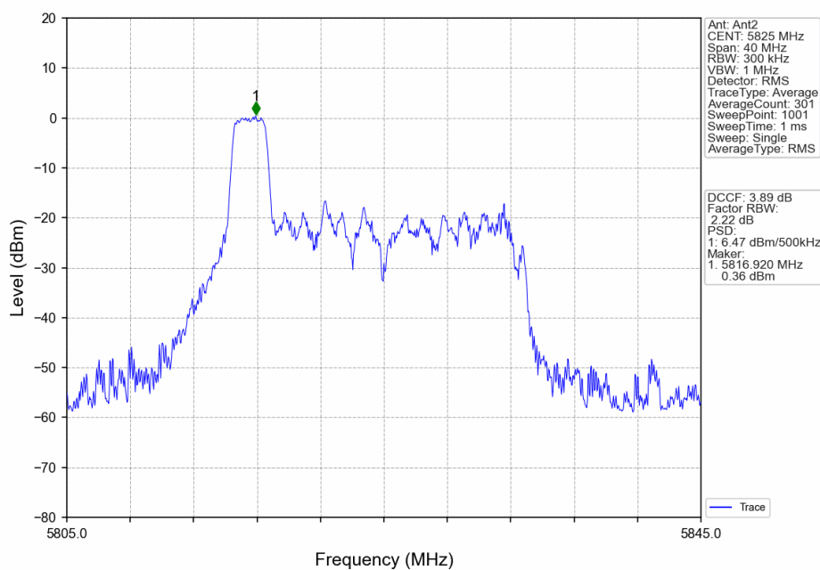
802.11ax(HEW20)_HCH_5825MHz_RU26_Left_Ant2_NTNV
