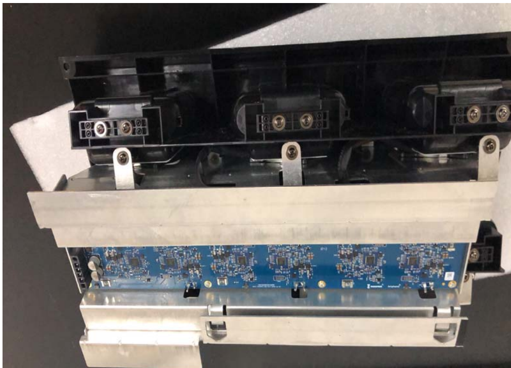
(24) EUT Photo
