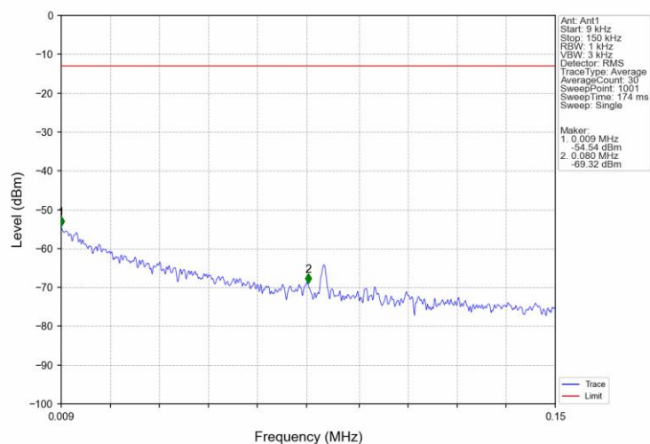
Band25 10MHz QPSK HCH 1910MHz RB 1 0 NTNV
