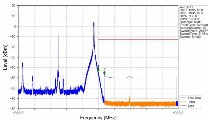
Band25 20MHz QPSK HCH 1905MHz RB 1 99 NTNV
