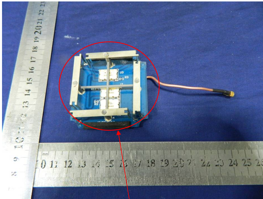
RFID Antenna
