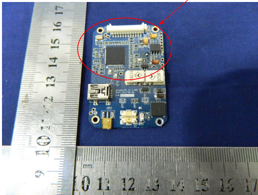
RFID module
