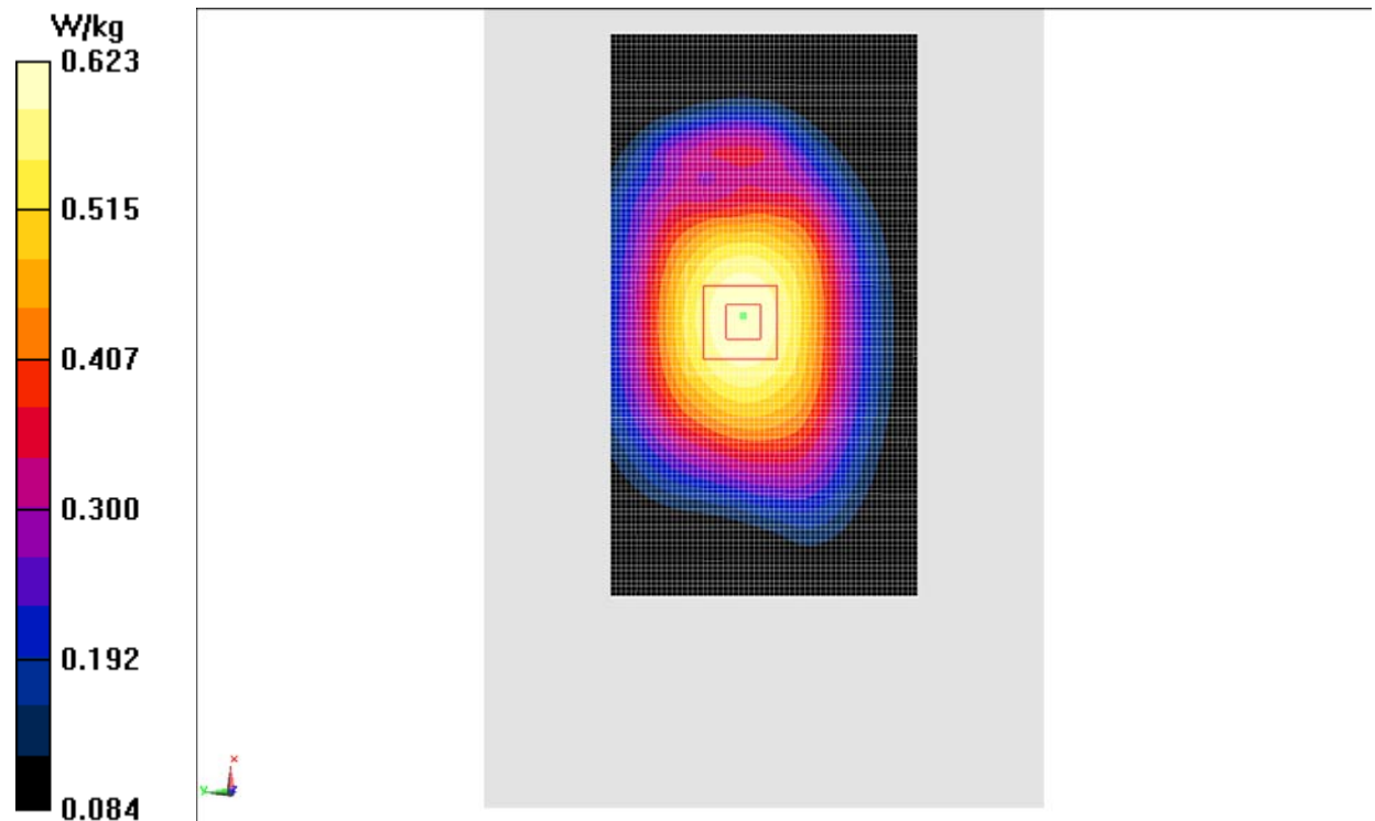
Fig.6 WCDMA 850
