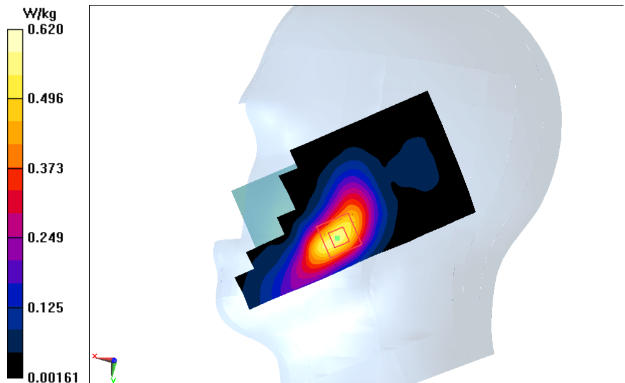
Fig.9 LTE Band7
