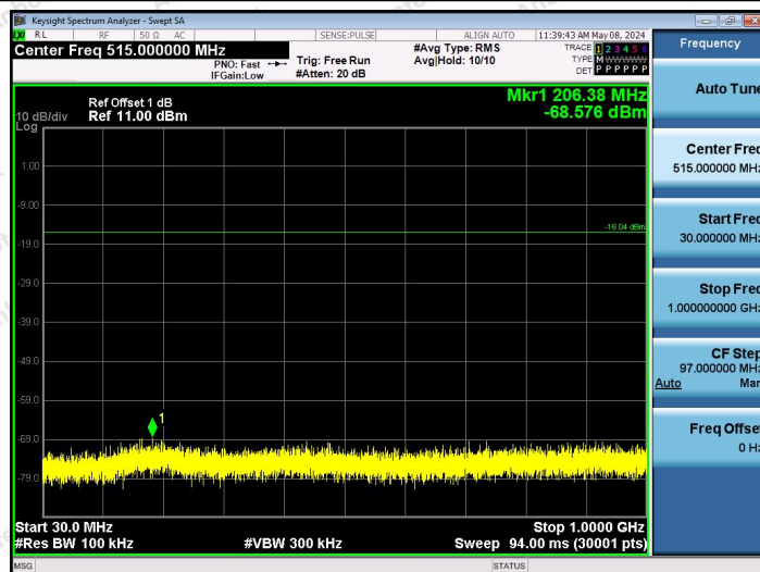
2.4G-Ant1-2403-30~1000-PASS
