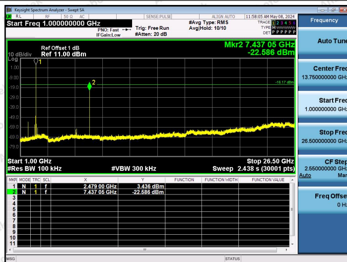
2.4G-Ant1-2479-1000~26500-PASS
