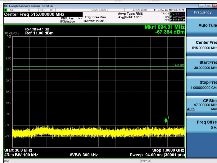
2.4G-Ant1-2479-30~1000-PASS
