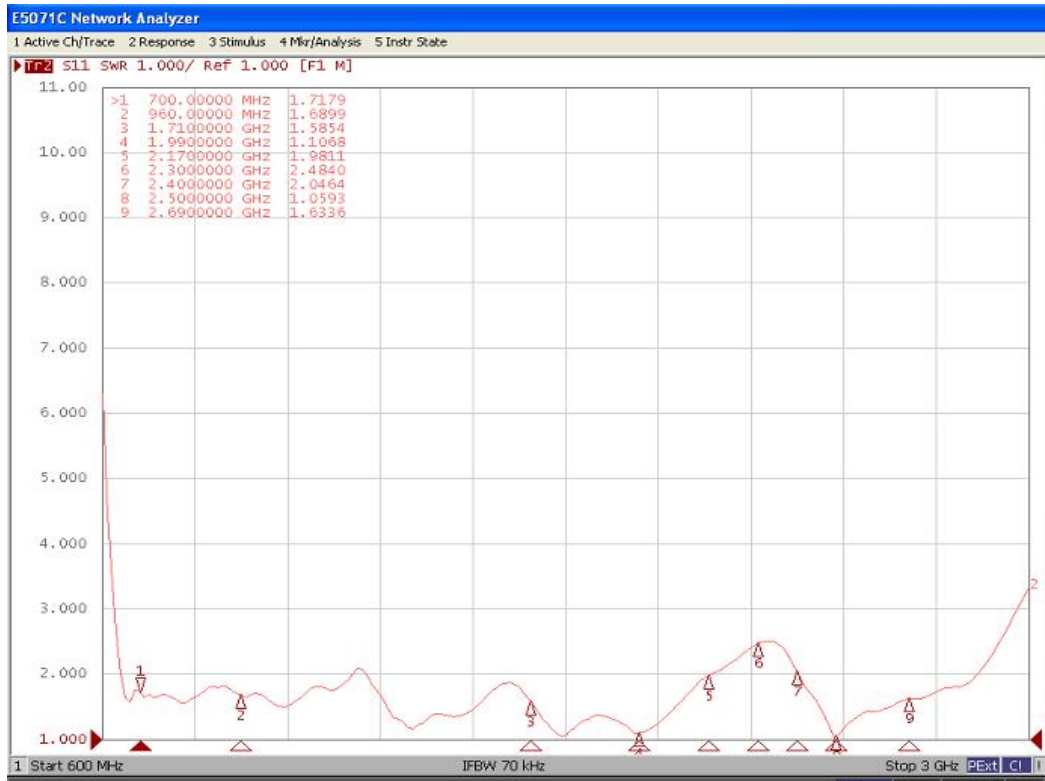
700~2700MHz antenna VSWR
