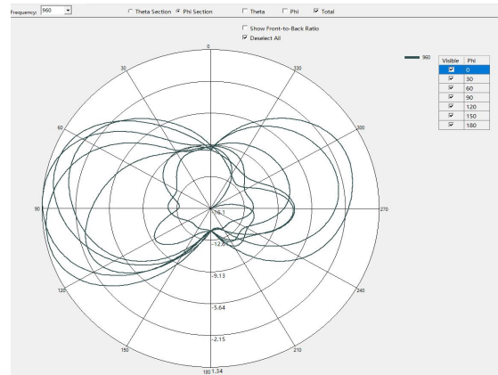
960MHz
