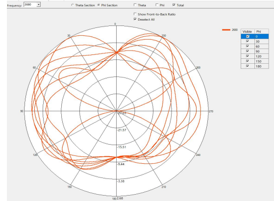
2680MHz
