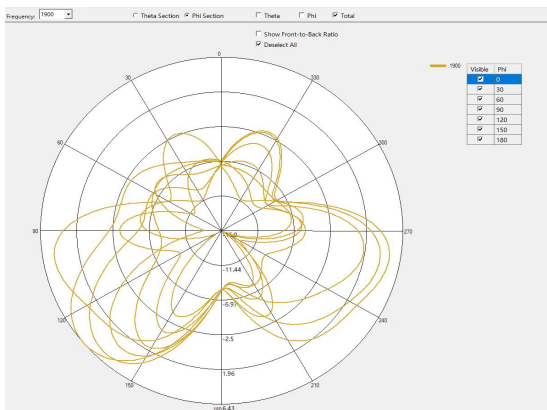
1900MHz
