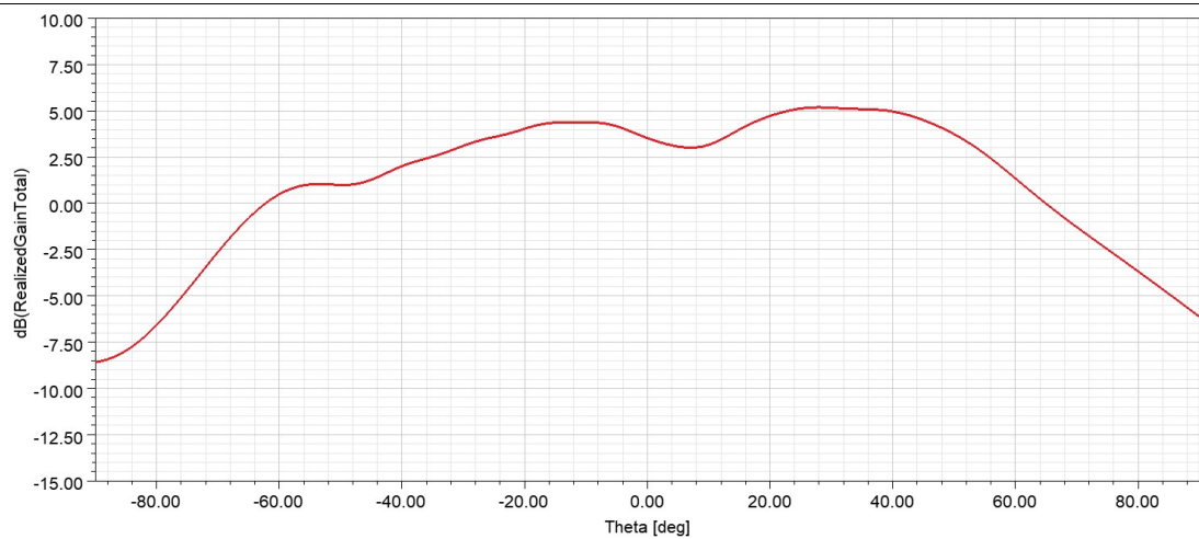
俯仰面方向图 (TX1) Freq: 60. 0GHz
