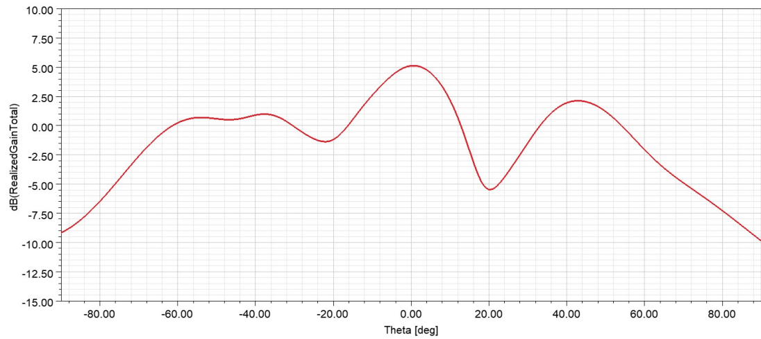
俯仰面向图 (TX0) Freq: 62. 0GHz
