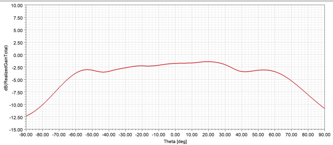
方位面方向图(TX1) Freq: 64. 0GHz
