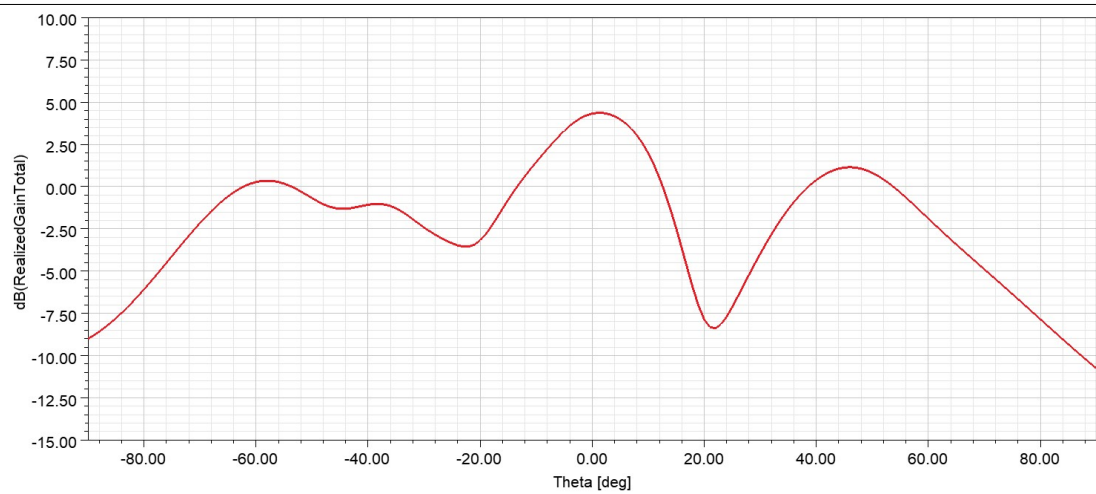
俯仰面方向图 (TX0) Freq: 63. 0GHz
