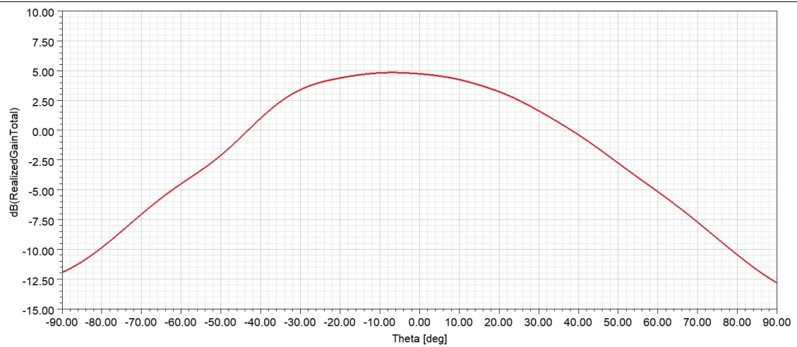
方位面方向图 (TX0) Freq: 59. 0GHz
