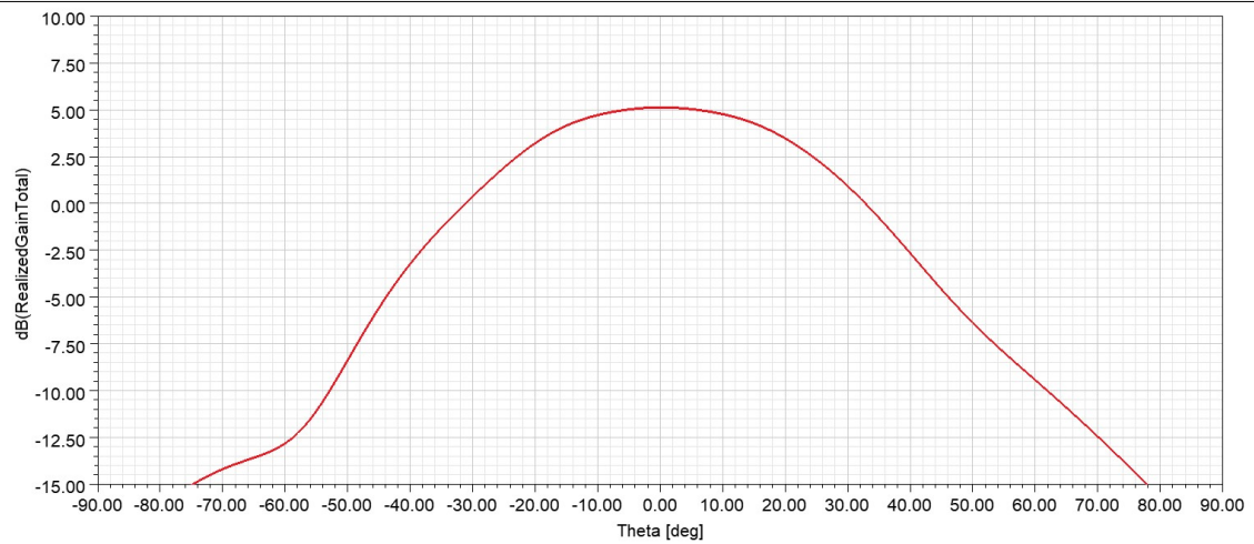
方位面方向图 (TX0) Freq: 63. 0GHz
