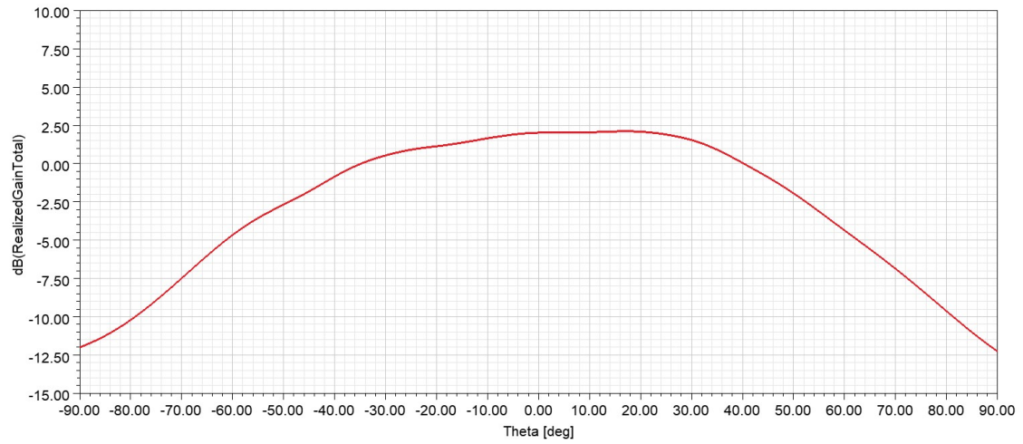
方位面方向图(TX1)Freq:61.0GHz
