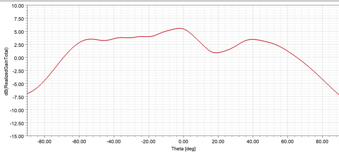
俯仰面方向图(TX0) Freq: 59 GHz
