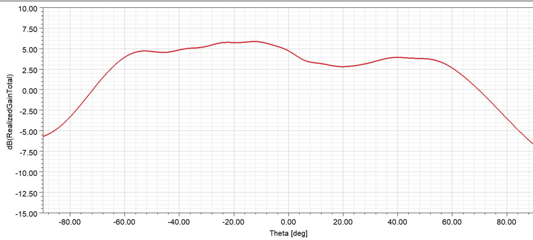
方位面方向图(TX1) Freq: 64. 0GHz
