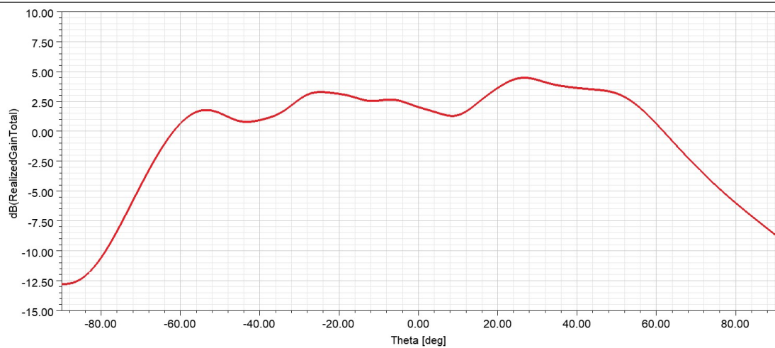
俯仰面方向图 (TX1) Freq: 61. 0GHz
