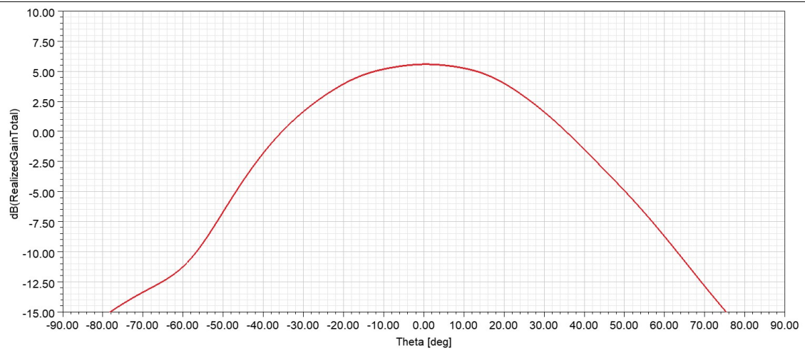
方位面方向图 (TX0) Freq: 61. 0GHz
