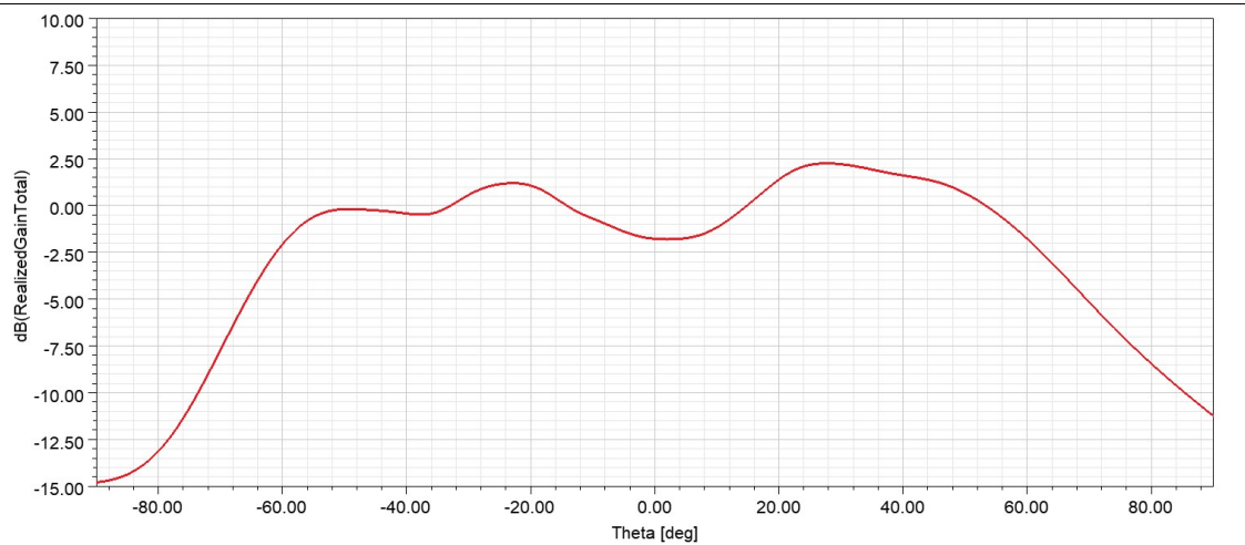
俯仰面方向图 (TX1) Freq: 63. 0GHz
