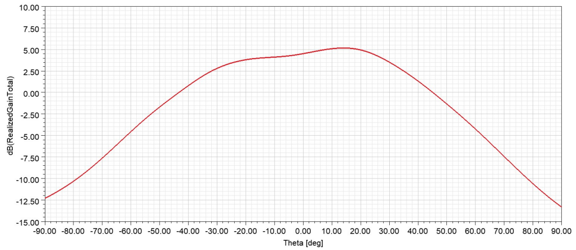
方位面方向图 (TX0) Freq: 64. 0GHz
