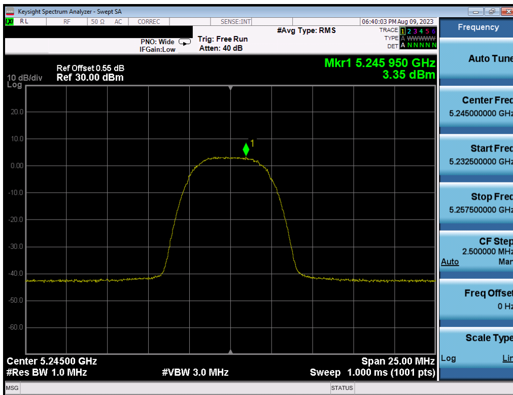
Plot 7-36. PSD (HDRp8, 5245MHz)
