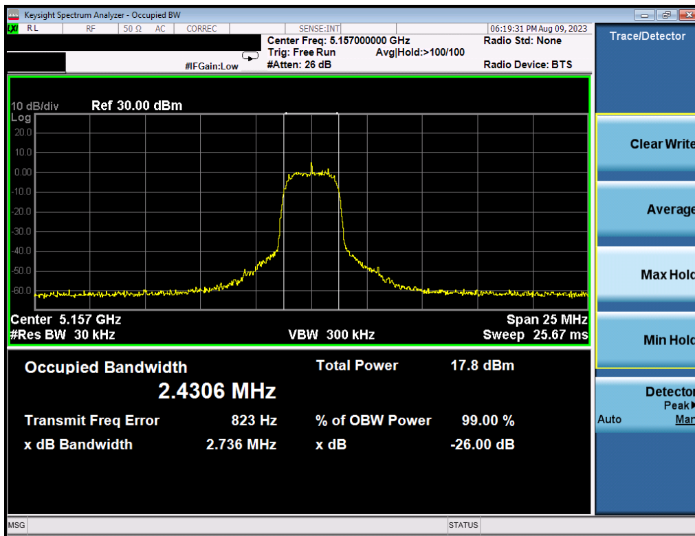
Plot 7-7. 26dB BW & 99% OBW (HDRp4, 5157MHz)
