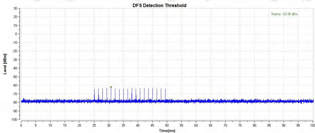
802.11n(HT20) SISO_5500_Type0
