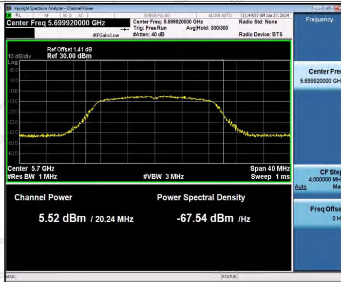
802.11n(HT20) SISO_Ant1_5700
