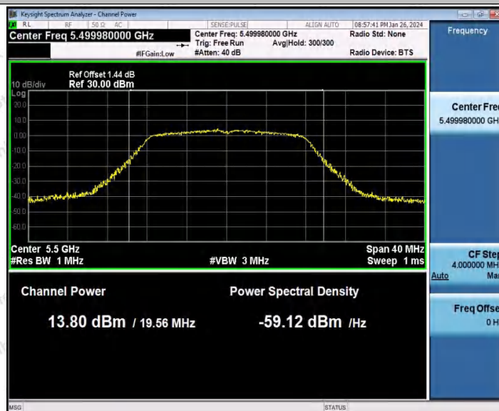
802.11a_Ant1_5500
