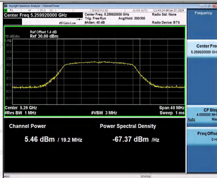
802.11a_Ant1_5260
