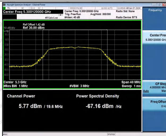
802.11a_Ant1_5300
