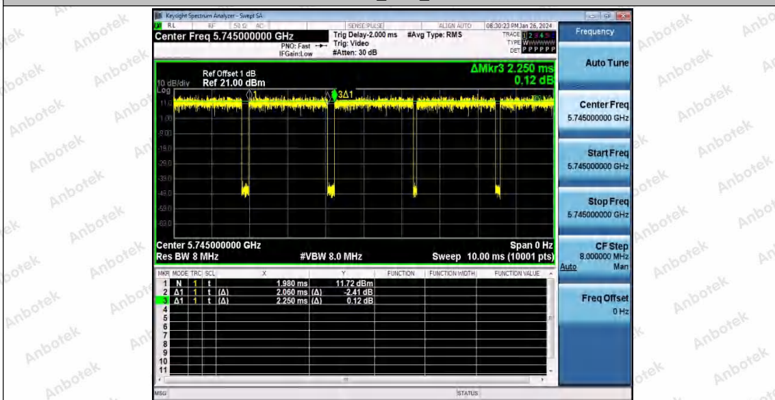
802.11a_Ant1_5745
