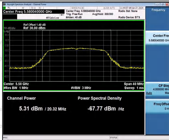
802.11n(HT20) SISO_Ant1_5580
