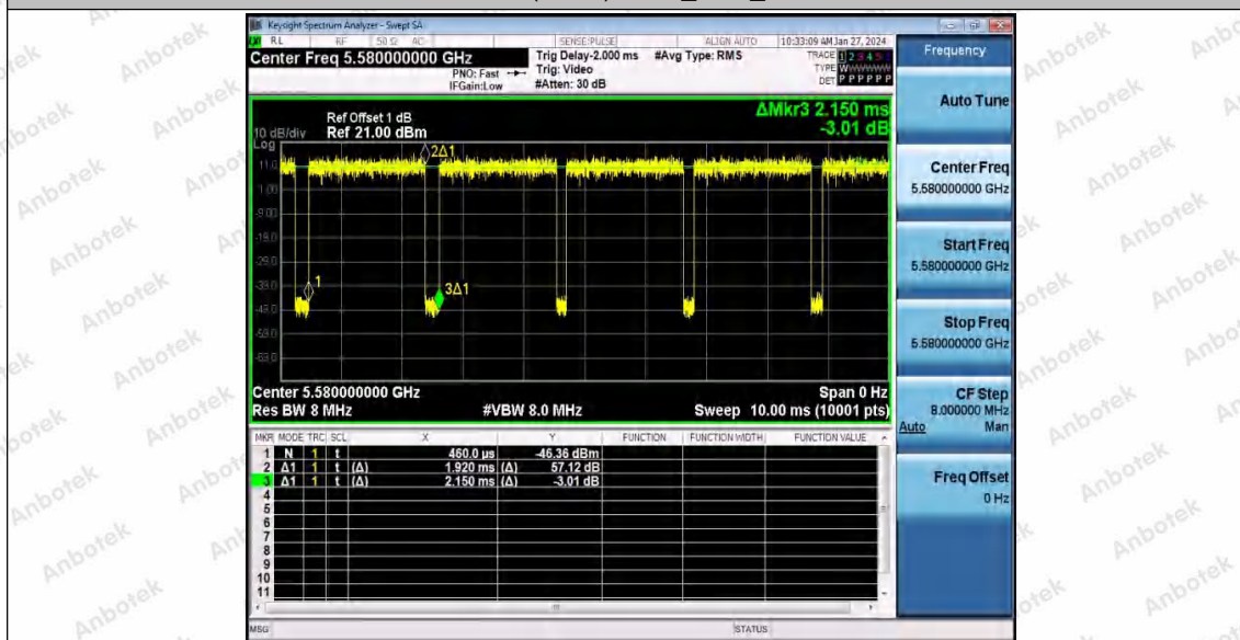
802.11n(HT20) SISO_Ant1_5580
