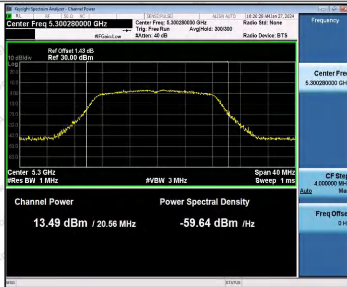
802.11n(HT20) SISO_Ant1_5300
