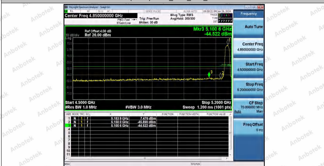
802.11n(HT20) SISO_Ant1_Low_5180
