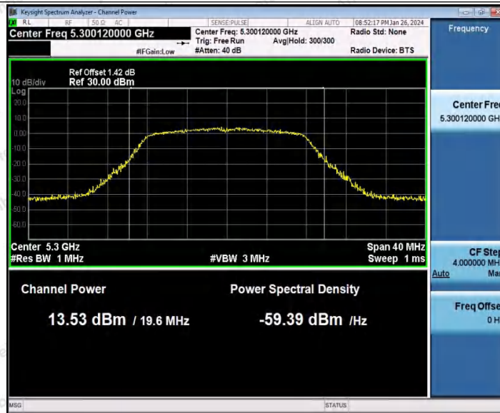
802.11a_Ant1_5300
