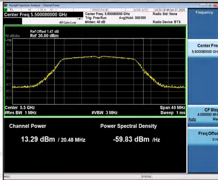
802.11n(HT20) SISO_Ant1_5500
