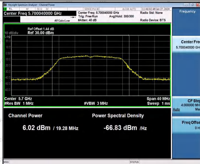
802.11a_Ant1_5700
