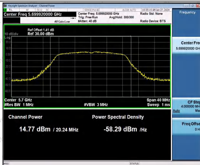
802.11n(HT20) SISO_Ant1_5700
