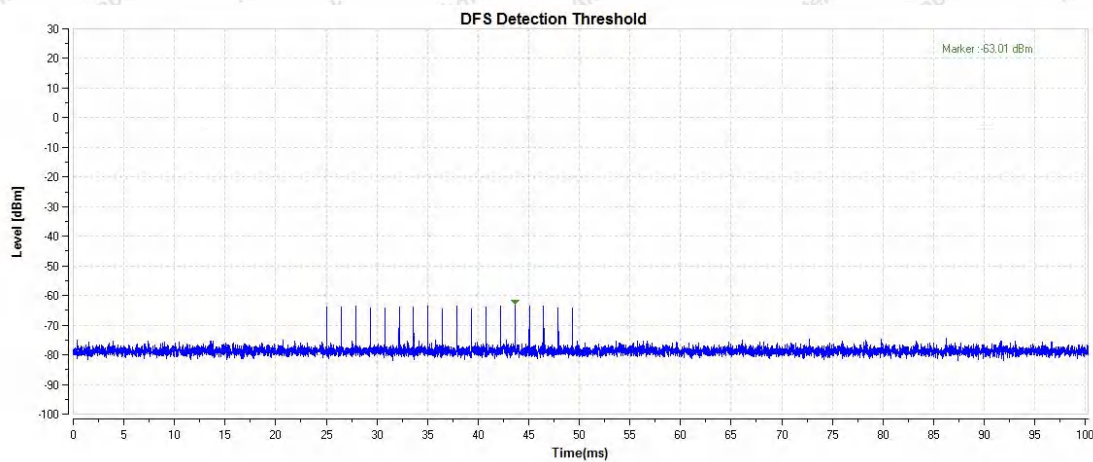
802.11n(HT20) SISO_5500_Type0
