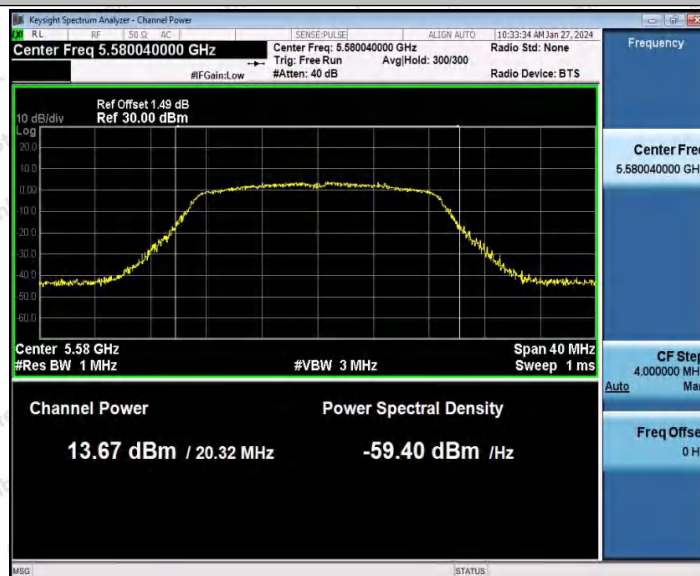
802.11n(HT20) SISO_Ant1_5580
