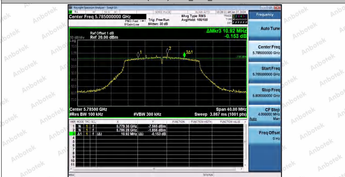
802.11n(HT20) SISO_Ant1_5785
