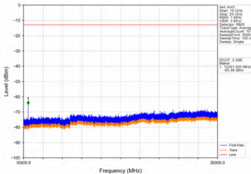
Band42a_10MHz_256QAM_LCH_3455MHz_RB_1_0_NTNV
