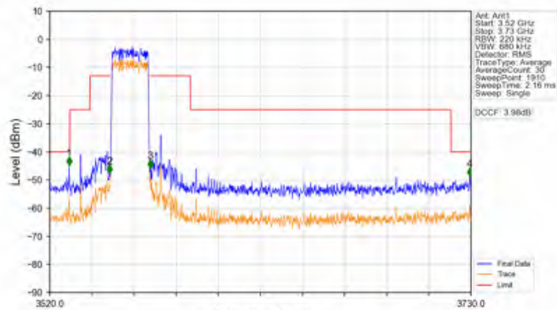
Band42c_20MHz_16QAM_LCH_3560MHz_RB_100_0_NTNV
