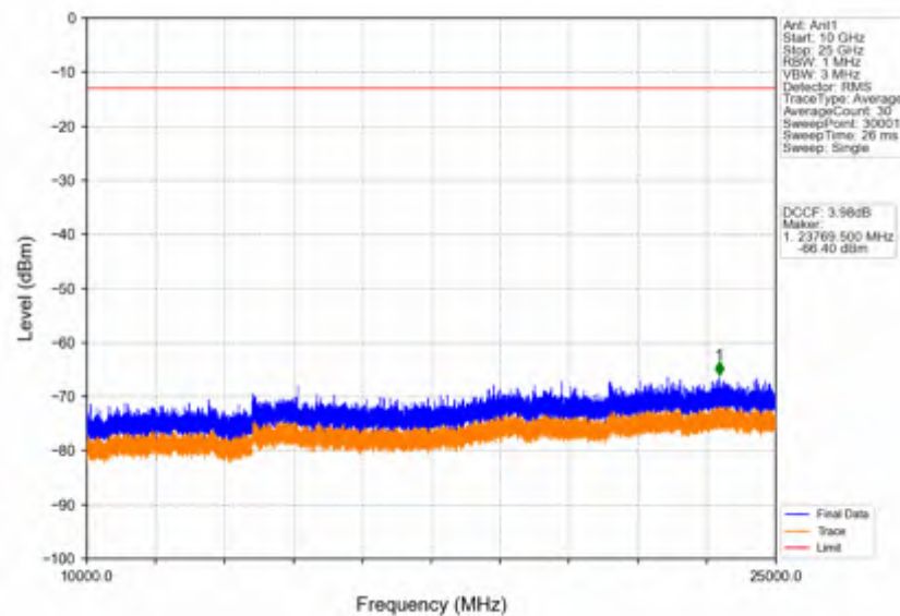
Band42c_20MHz_QPSK_MCH_3575MHz_RB_1_0_NTNV
