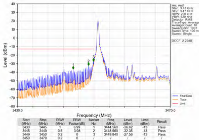
Band42a_20MHz_QPSK_LCH_3460MHz_RB_1_0_NTNV
