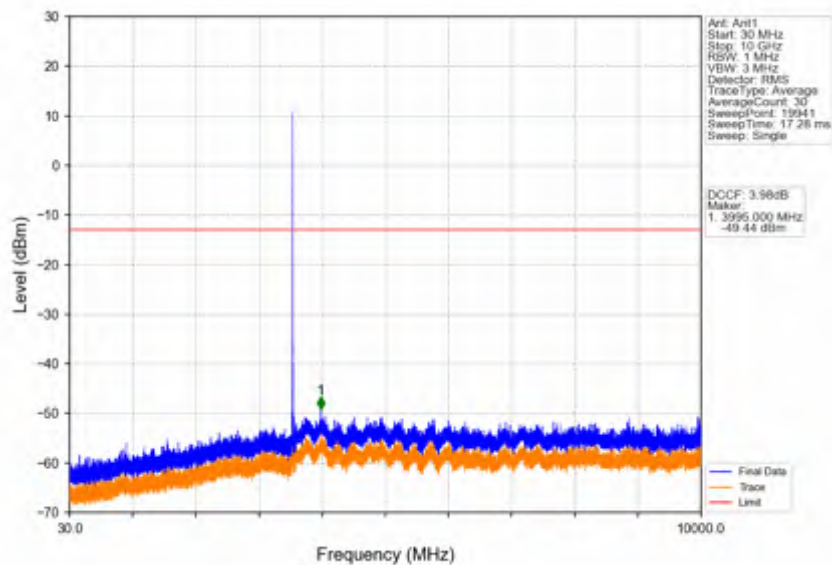
Band42c_10MHz_256QAM_LCH_3555MHz_RB_1_0_NTNV
