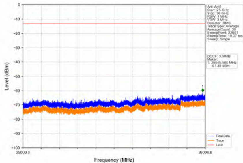
Band42c_10MHz_QPSK_LCH_3555MHz_RB_1_0_NTNV
