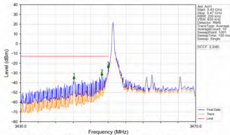
Band42a_20MHz_16QAM_LCH_3460MHz_RB_100_0_NTNV
