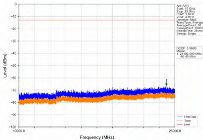
Band42c_10MHz_16QAM_LCH_3555MHz_RB_1_0_NTNV
