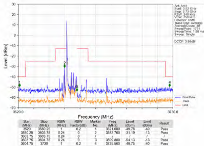
Band42c_15MHz_QPSK_HCH_3592.5MHz_RB_1_74_NTNV
