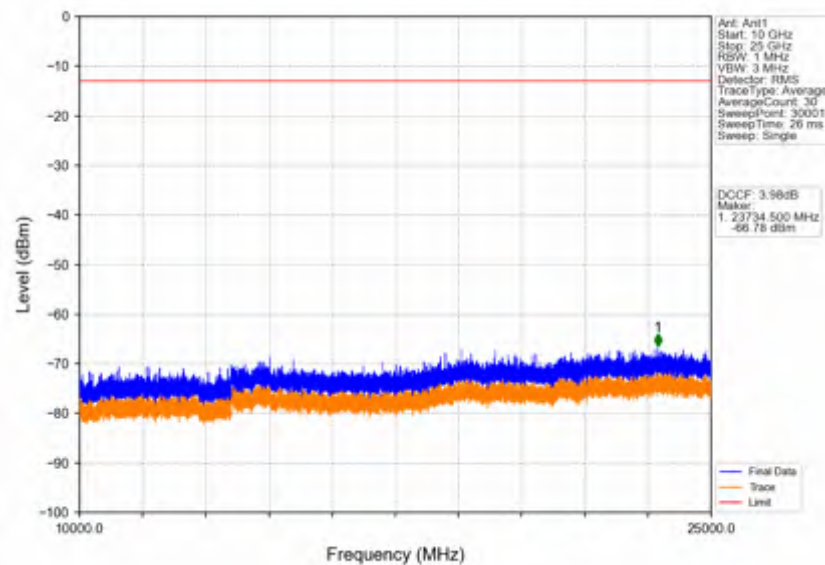
Band42c_10MHz_QPSK_MCH_3575MHz_RB_1_0_NTNV
