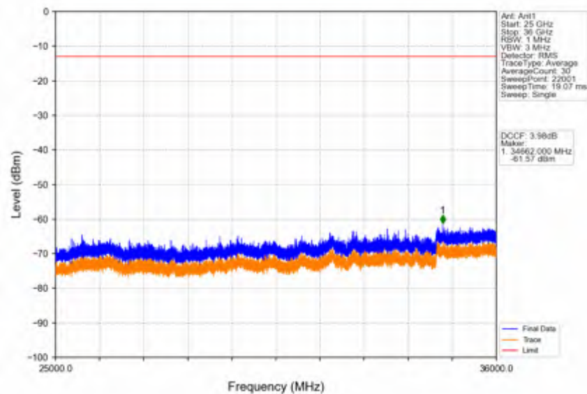
Band42c_15MHz_QPSK_HCH_3592.5MHz_RB_1_74_NTNV
