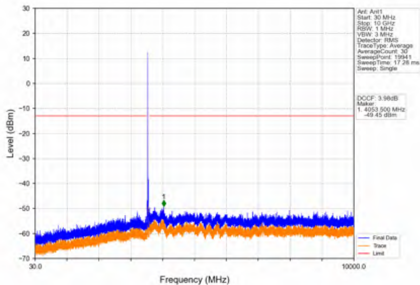
Band42c_20MHz_16QAM_LCH_3560MHz_RB_1_0_NTNV
