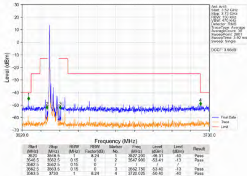
Band42c_10MHz_QPSK_LCH_3555MHz_RB_1_0_NTNV
