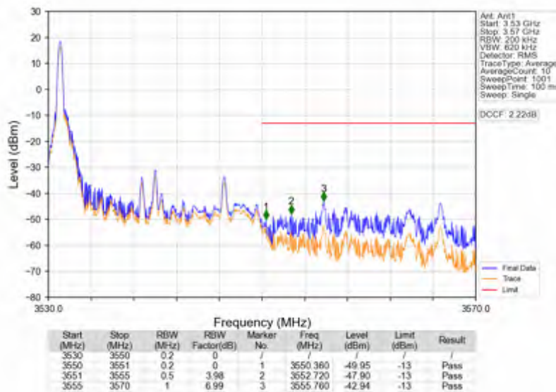
Band42a_20MHz_QPSK_HCH_3540MHz_RB_1_99_NTNV
