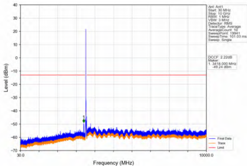
Band42a_20MHz_QPSK_HCH_3540MHz_RB_1_0_NTNV
