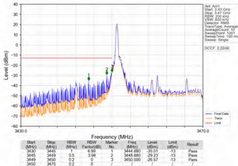
Band42a_20MHz_QPSK_LCH_3460MHz_RB_100_0_NTNV
