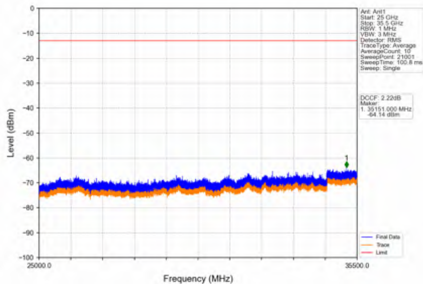
Band42a_20MHz_256QAM_LCH_3460MHz_RB_100_0_NTNV
