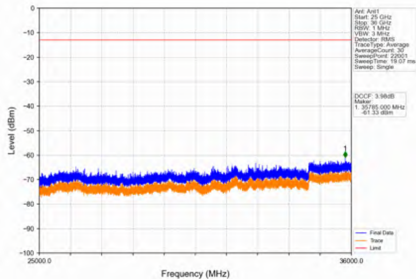
Band42c_10MHz_QPSK_MCH_3575MHz_RB_1_0_NTNV
