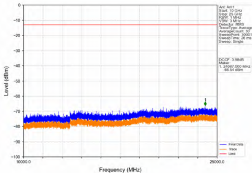
Band42c_10MHz_QPSK_HCH_3595MHz_RB_1_0_NTV
