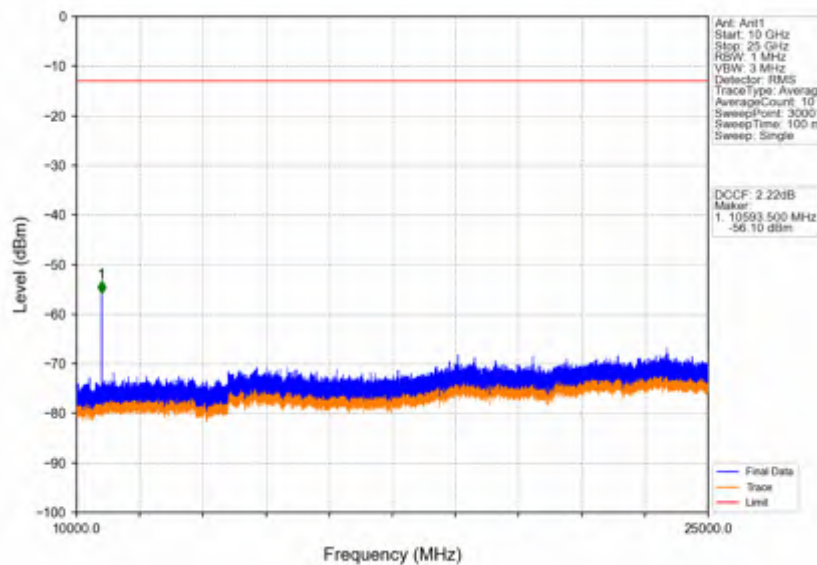
Band42a_20MHz_QPSK_HCH_3540MHz_RB_1_0_NTNV
