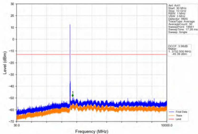
Band42c_20MHz_QPSK_HCH_3590MHz_RB_1_0_NTNV
