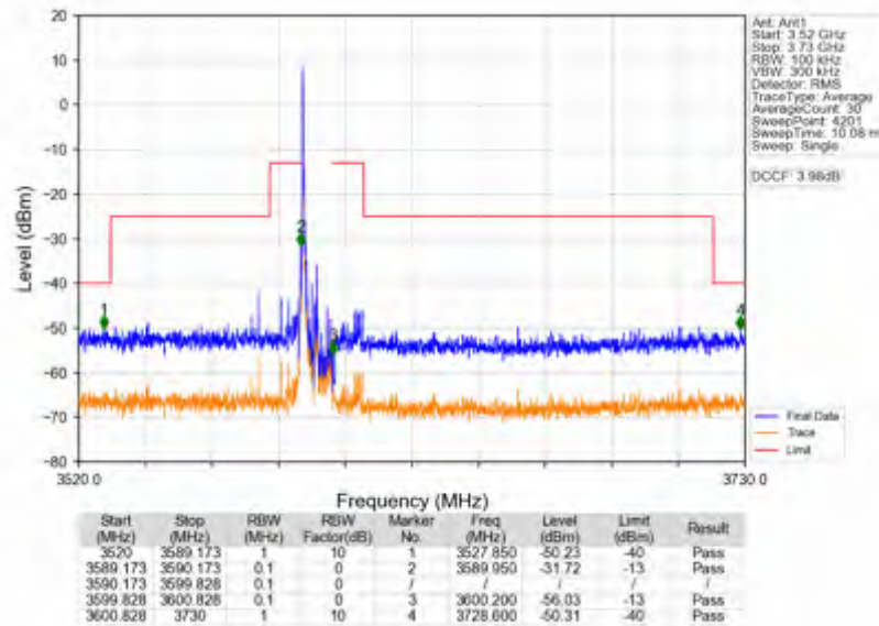
Band42c_10MHz_256QAM_LCH_3555MHz_RB_1_0_NTNV
