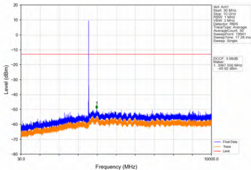
Band42c_10MHz_QPSK_MCH_3575MHz_RB_1_0_NTNV
