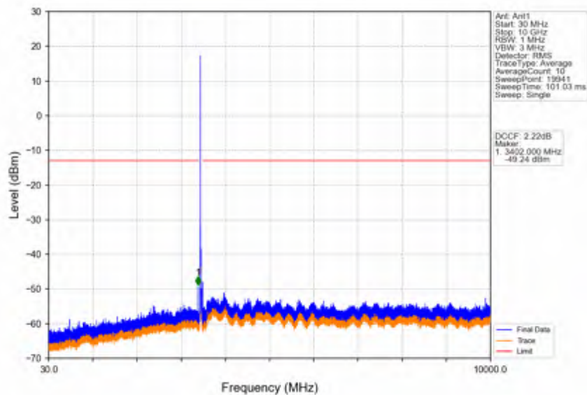
Band42a_20MHz_256QAM_LCH_3460MHz_RB_1_0_NTNV
