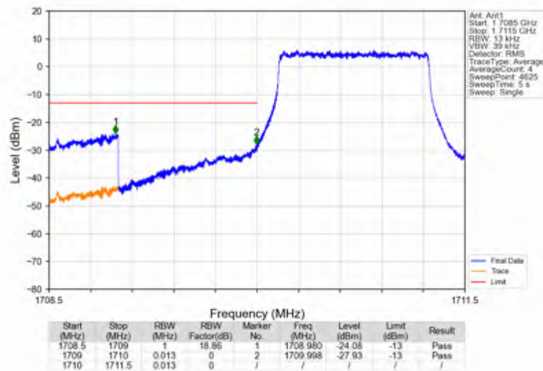
Band66 1.4MHz QPSK LCH 1710.7MHz RB 6 0 NTNV
