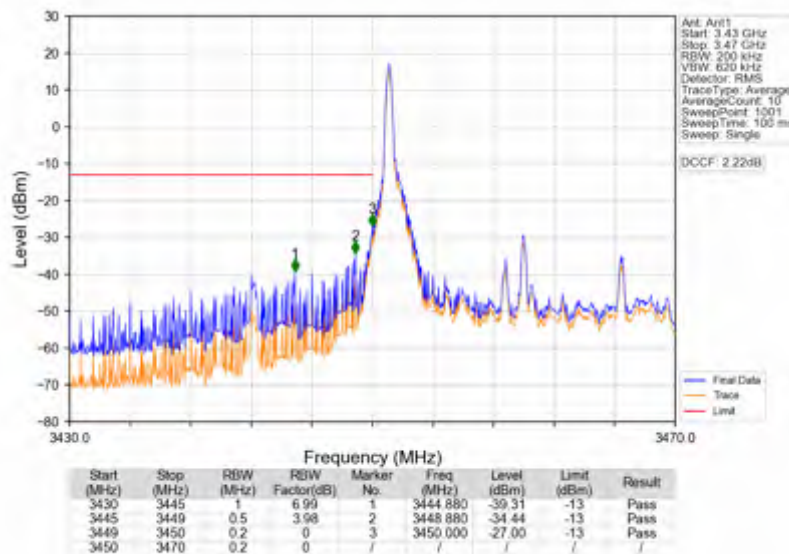
Band42a_20MHz_256QAM_LCH_3460MHz_RB_1_0_NTNV
