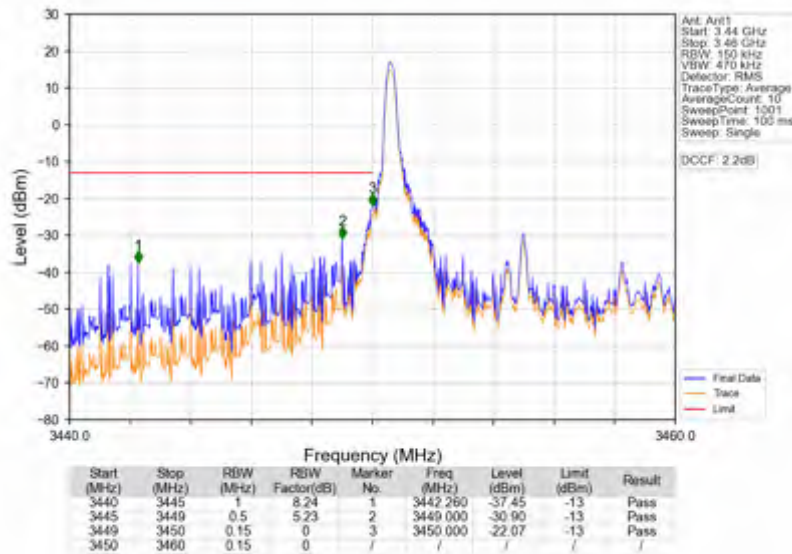
Band42a_10MHz_256QAM_LCH_3455MHz_RB_1_0_NTNV
