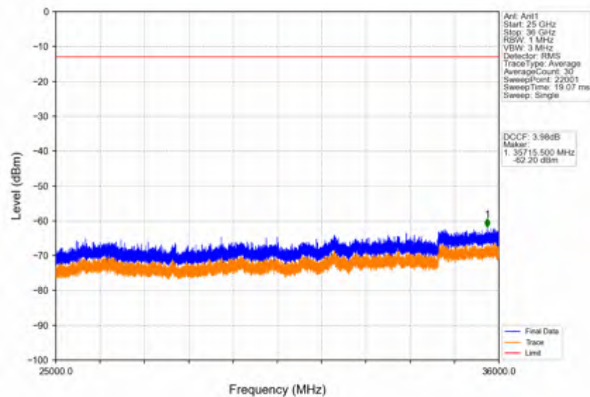
Band42c_20MHz_QPSK_HCH_3590MHz_RB_1_99_NTNV
