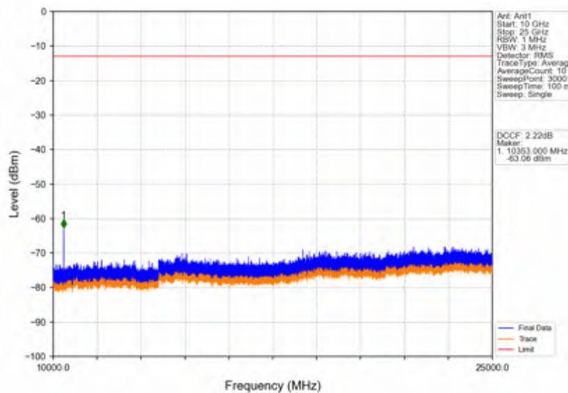
Band42a_20MHz_256QAM_LCH_3460MHz_RB_1_0_NTNV
