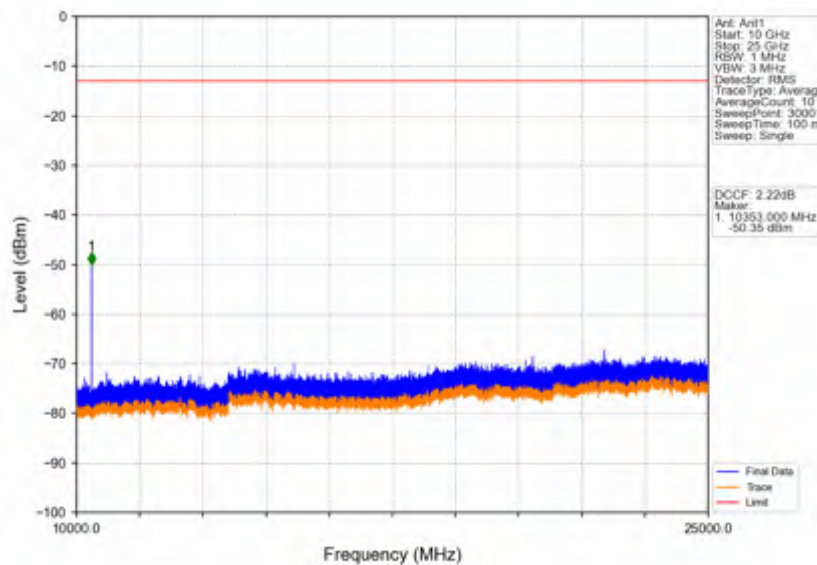
Band42a_20MHz_16QAM_LCH_3460MHz_RB_1_0_NTNV
