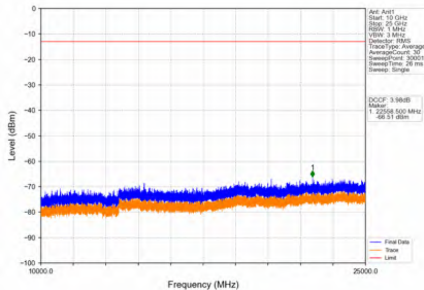
Band42c_20MHz_QPSK_LCH_3560MHz_RB_1_0_NTNV
