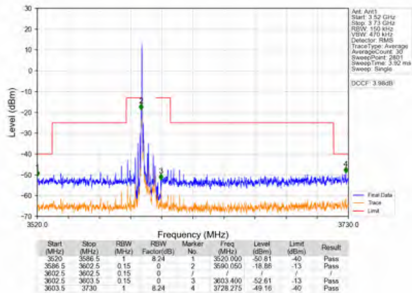
Band42c_10MHz_QPSK_HCH_3595MHz_RB_1_49_NTNV
