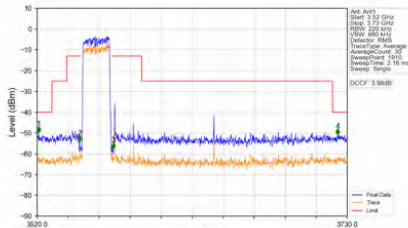
Band42c_20MHz_256QAM_LCH_3560MHz_RB_100_0_NTNV
