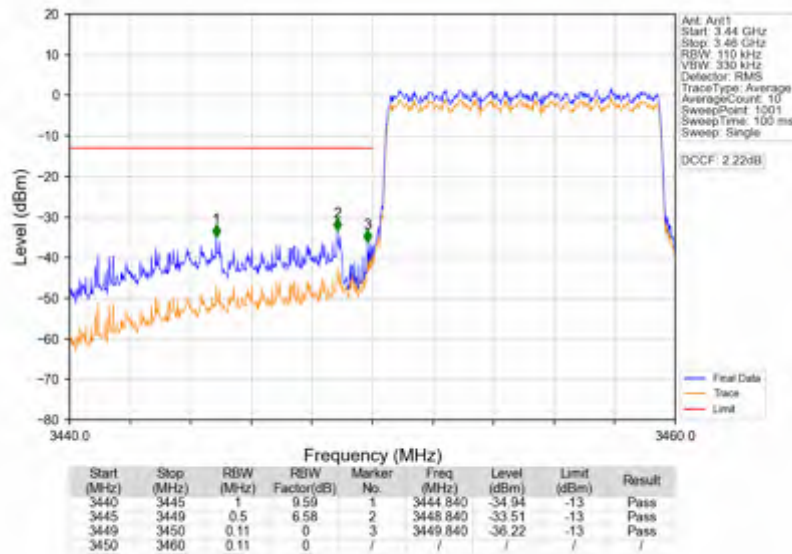
Band42a_10MHz_256QAM_LCH_3455MHz_RB_50_0_NTNV
