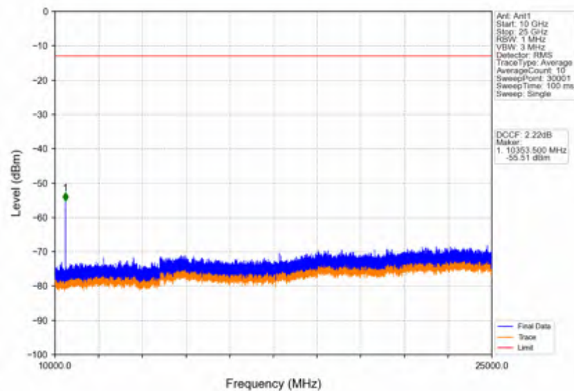
Band42a 20MHz 64QAM LCH 3460MHz RB 1 0 NTV
