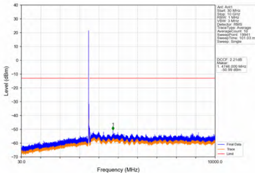
Band42a_20MHz_QPSK_MCH_3500MHz_RB_1_0_NTNV
