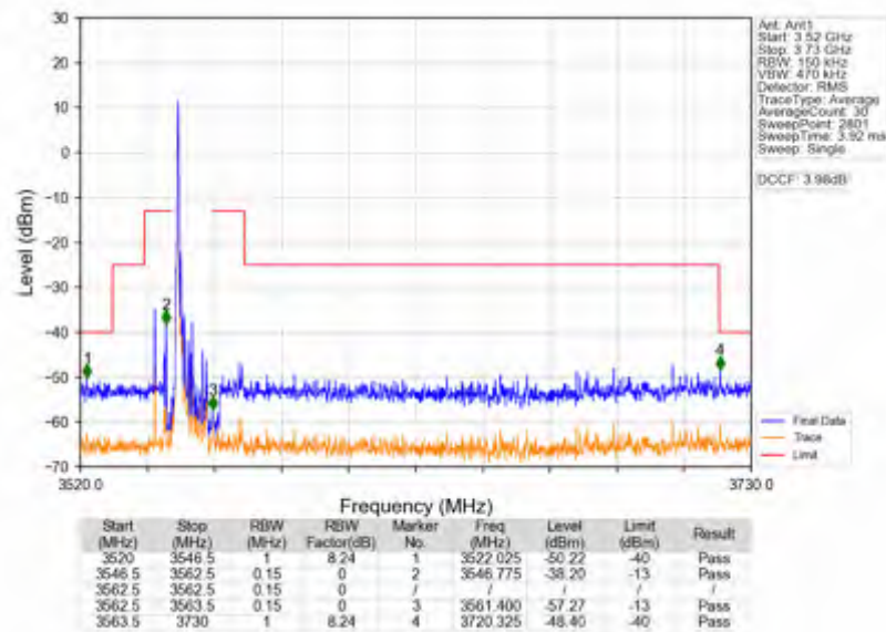
Band42c_10MHz_16QAM_LCH_3555MHz_RB_1_0_NTNV
