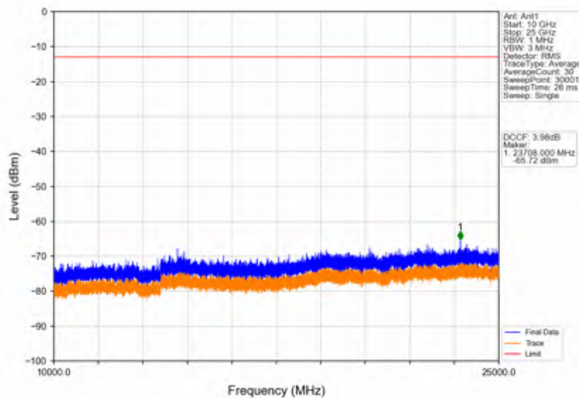
Band42c_20MHz_16QAM_LCH_3560MHz_RB_1_0_NTNV
