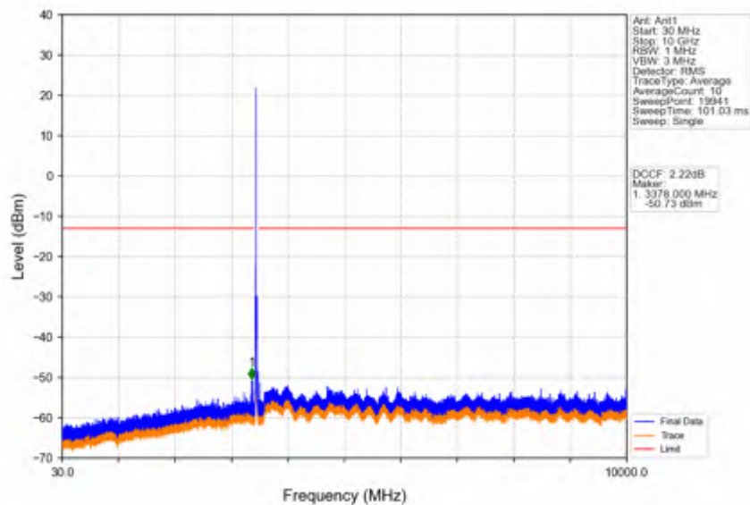
Band42a_20MHz_16QAM_LCH_3460MHz_RB_1_0_NTNV
