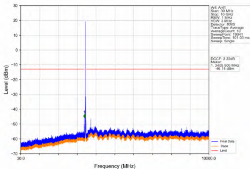
Band42a_20MHz_QPSK_LCH_3460MHz_RB_1_0_NTNV
