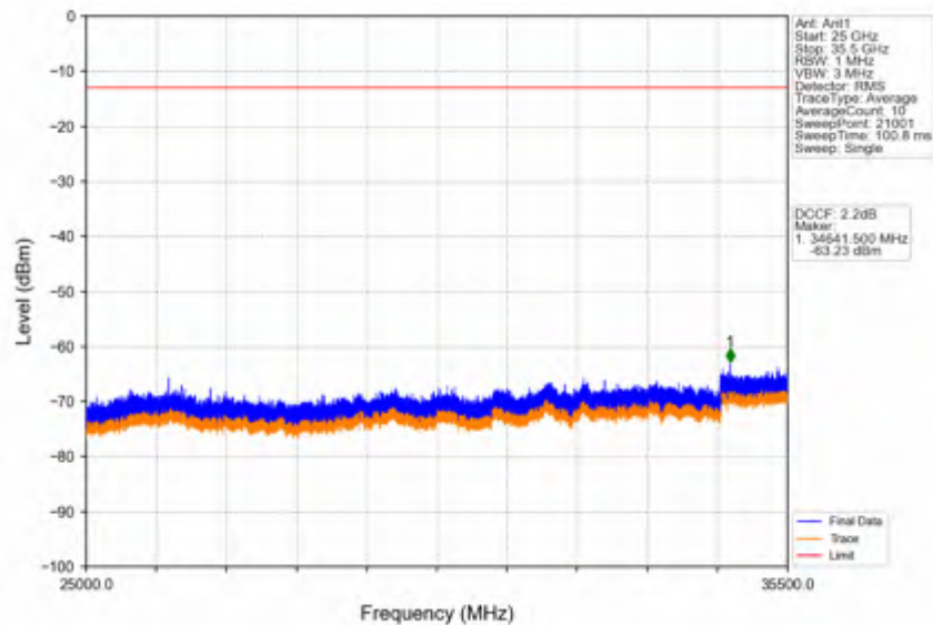
Band42a_10MHz_256QAM_LCH_3455MHz_RB_50_0_NTNV
