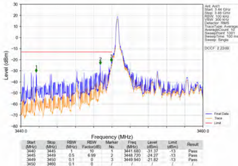
Band42a 10MHz 64QAM LCH 3455MHz RB 50 0 NTNV
