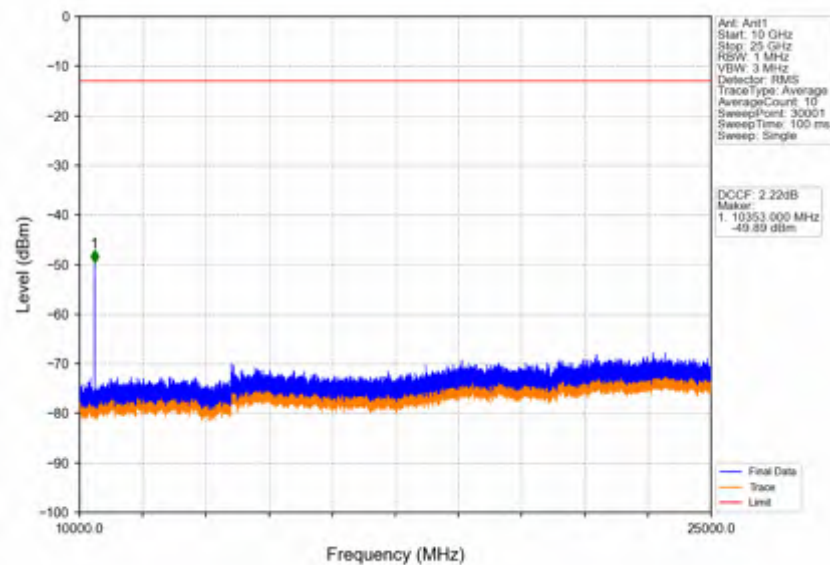
Band42a_20MHz_QPSK_LCH_3460MHz_RB_1_0_NTNV
