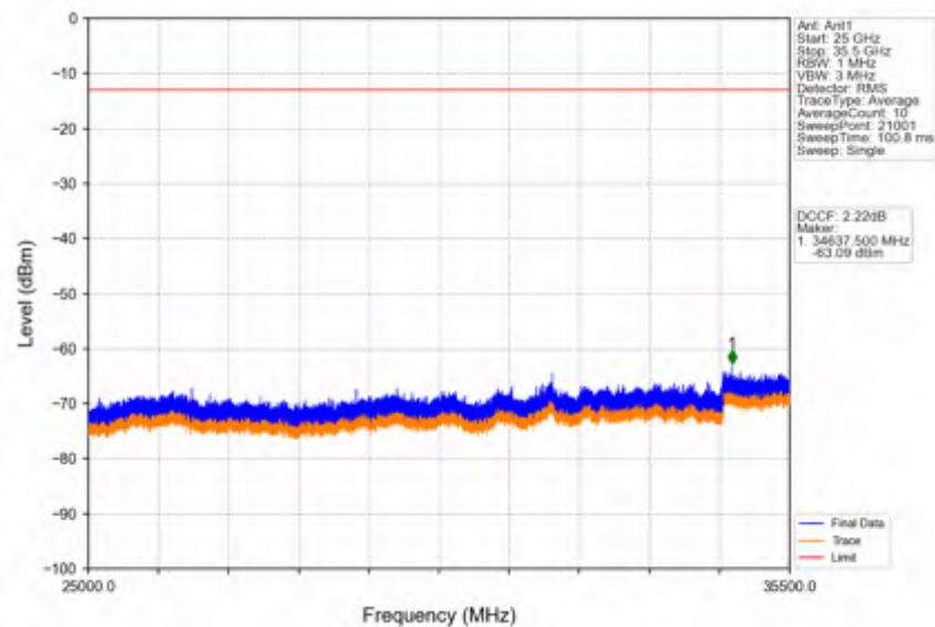
Band42a_20MHz_QPSK_LCH_3460MHz_RB_1_0_NTNV
