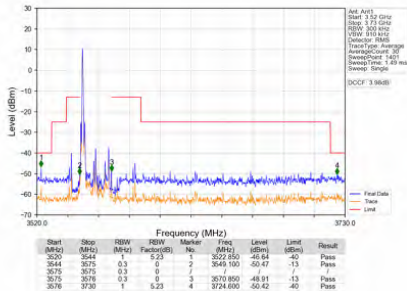
Band42c_20MHz_16QAM_LCH_3560MHz_RB_1_0_NTNV
