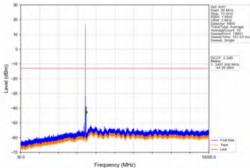
Band42a_10MHz_256QAM_LCH_3455MHz_RB_1_0_NTNV
