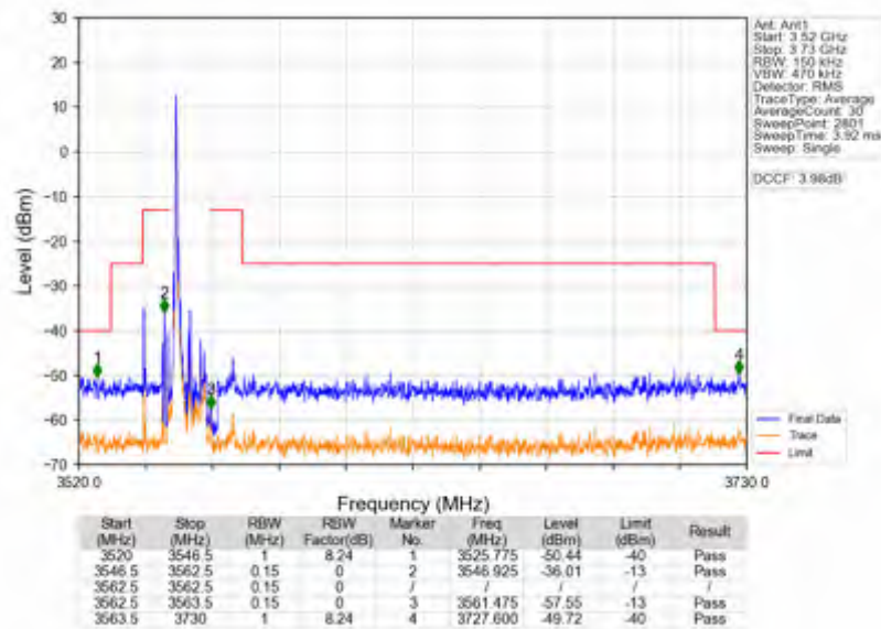
Band42c_10MHz_256QAM_LCH_3555MHz_RB_1_0_NTNV
