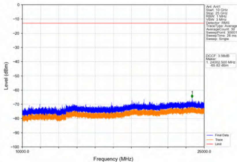
Band42c_10MHz_256QAM_LCH_3555MHz_RB_1_0_NTNV
