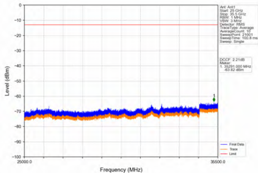
Band42a_20MHz_QPSK_MCH_3500MHz_RB_1_0_NTNV
