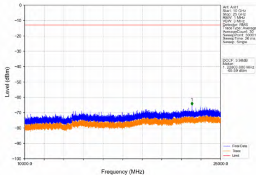
Band42c_10MHz_QPSK_LCH_3555MHz_RB_1_0_NTNV
