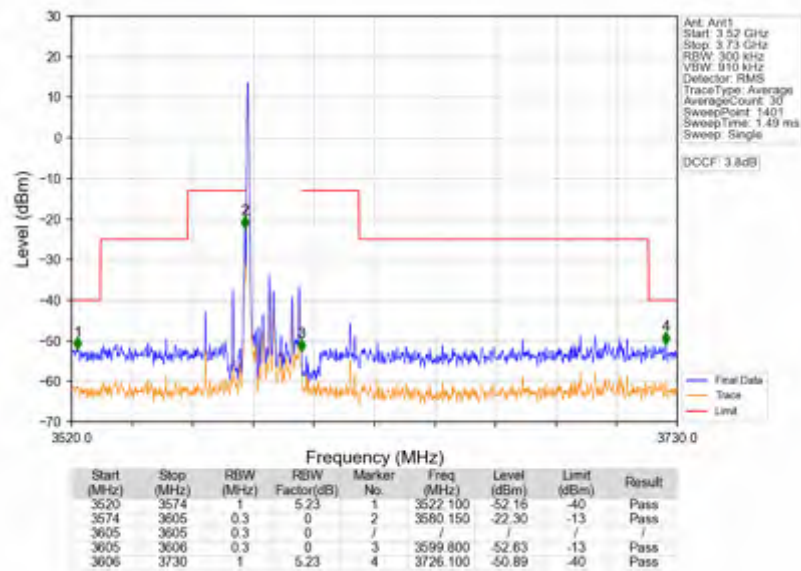
Band42c_20MHz_QPSK_HCH_3590MHz_RB_1_99_NTNV
