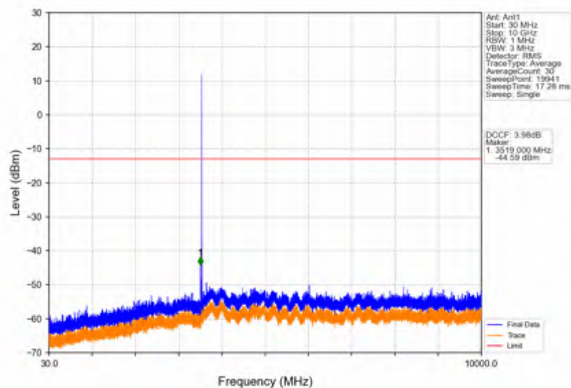
Band42c_10MHz_QPSK_LCH_3555MHz_RB_1_0_NTNV
