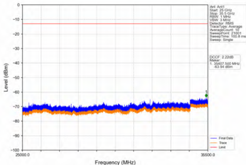
Band42a_20MHz_QPSK_HCH_3540MHz_RB_1_99_NTNV
