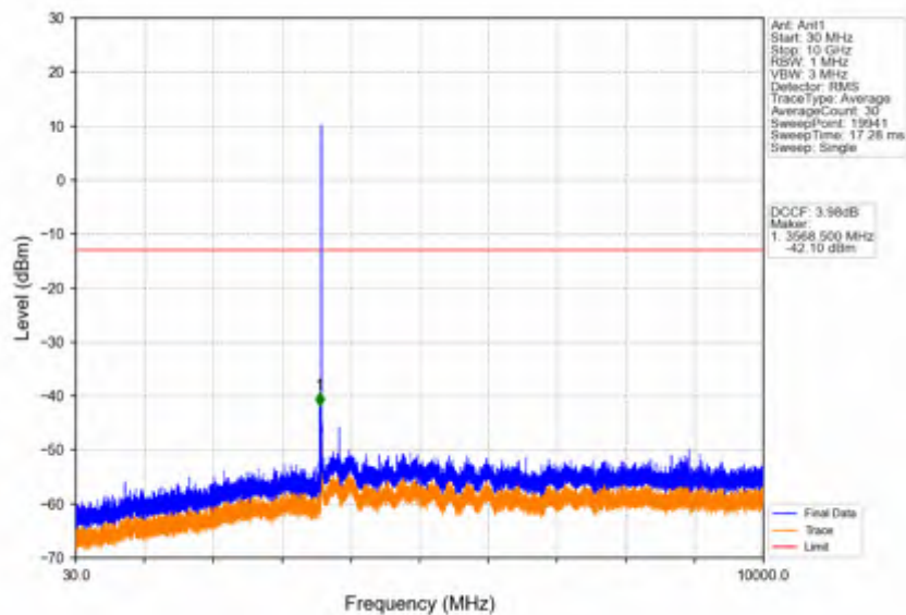
Band42c_10MHz_QPSK_HCH_3595MHz_RB_1_0_NTV
