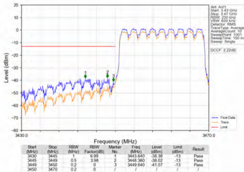
Band42a_20MHz_256QAM_LCH_3460MHz_RB_100_0_NTNV
