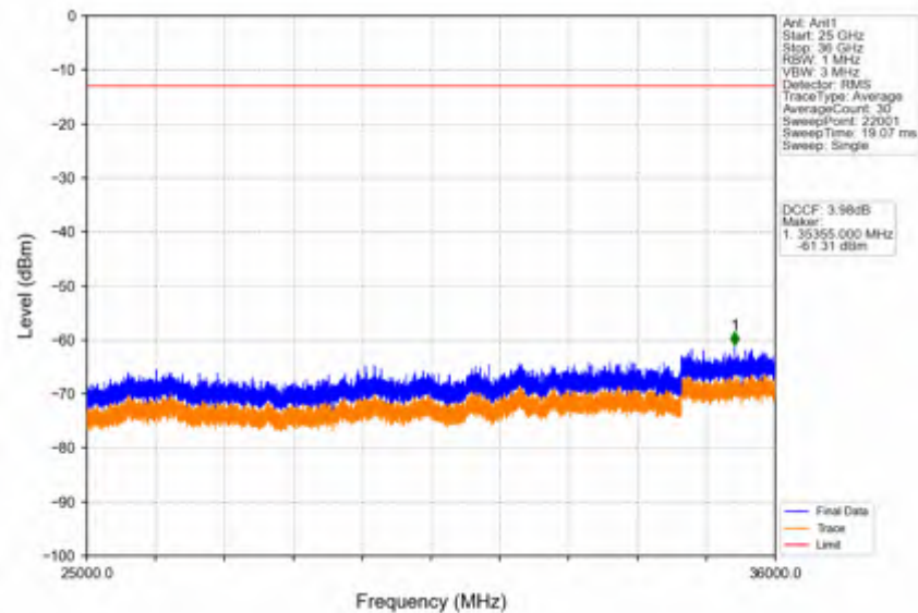
Band42c_10MHz_QPSK_HCH_3595MHz_RB_1_49_NTNV
