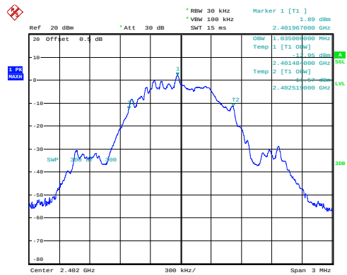
Low 1.035MHz
