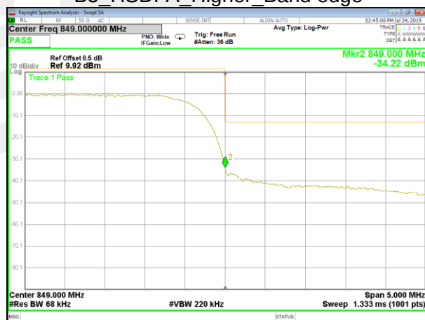
B5_HSUPA_Higher_Band edge
