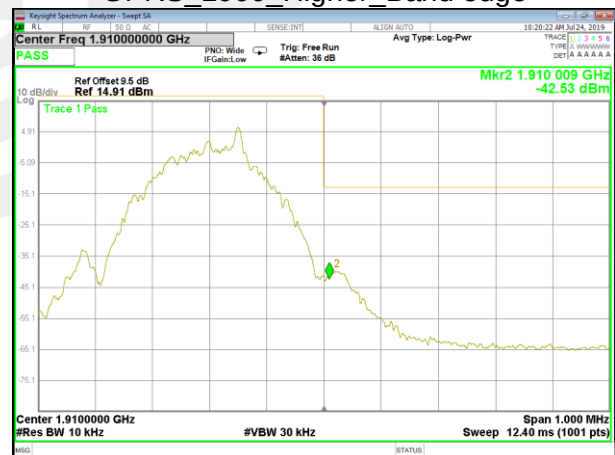
EGPRS_1900_Higher_Band edge
