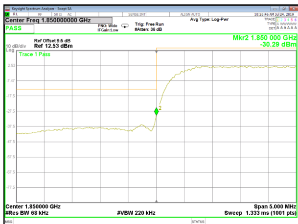
B2_WCDMA_Lower_Band edge
