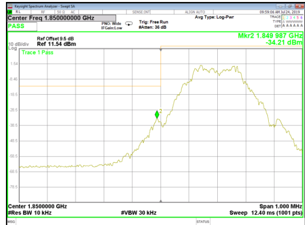
GPRS_1900_Lower_Band edge
