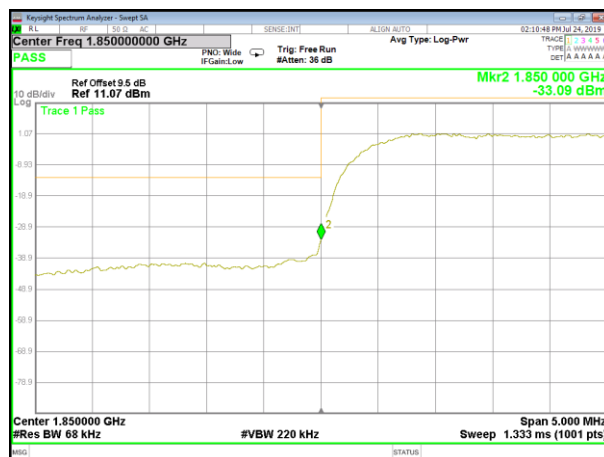
B2_HSDPA_Lower_Band edge
