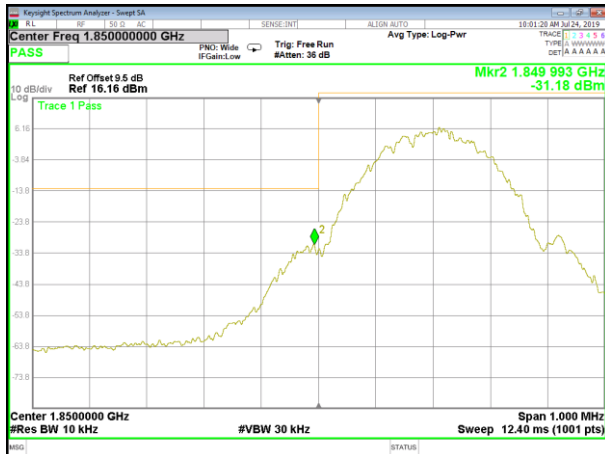
GSM_1900_Lower_Band edge
