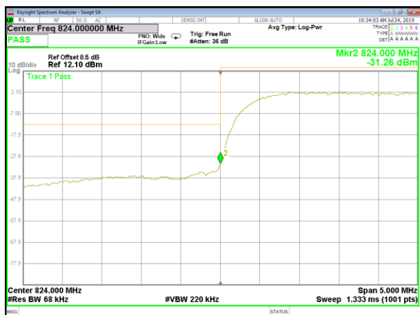
B5_WCDMA_Lower_Band edge
