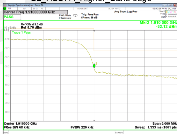
B2_HSUPA_Higher_Band edge
