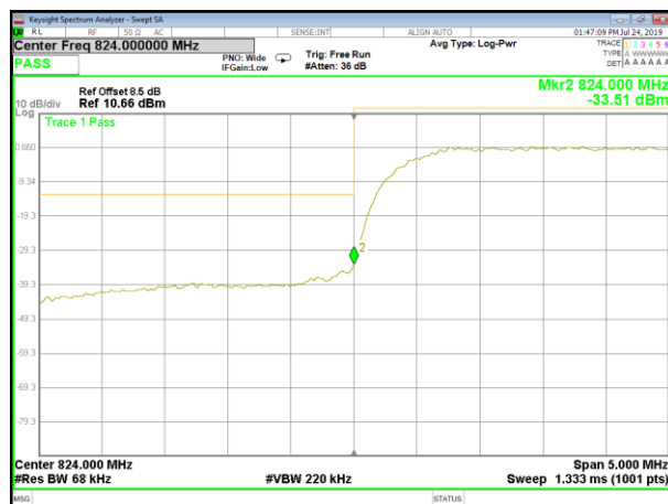
B5_HSDPA_Lower_Band edge
