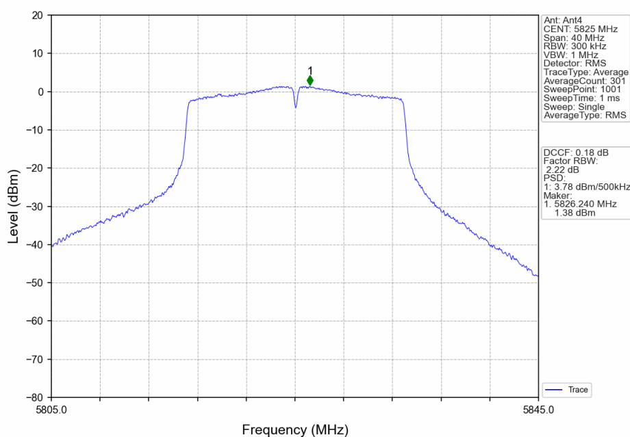
802.11n(HT20)_HCH_5825MHz_Ant4_NTNV
