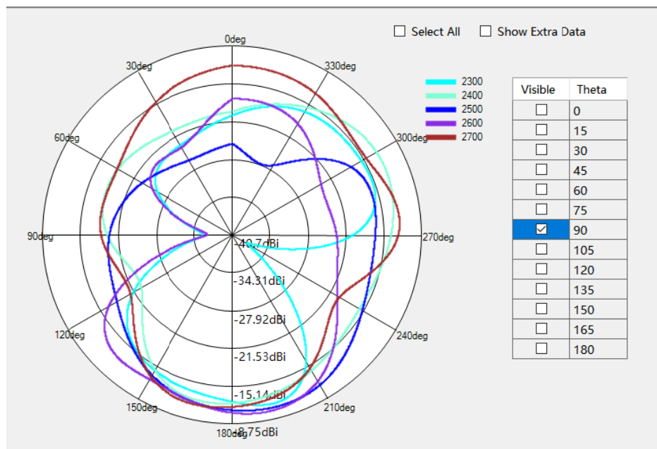
LTE B7/38/40/41 Theta=90deg
