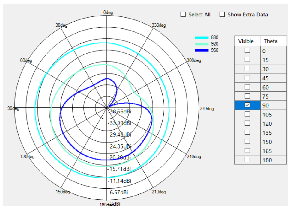
GSM900/WCDMA B8/LTE B8 Theta=90deg
