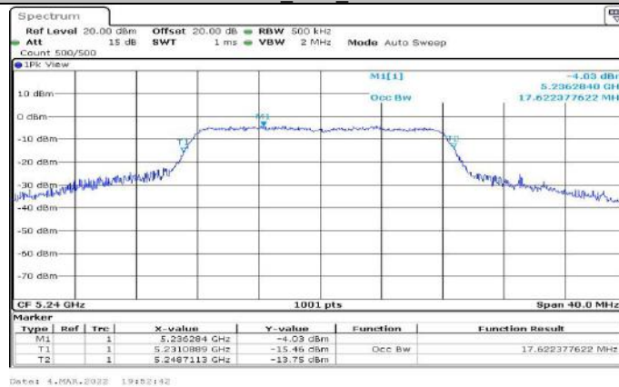
11A_Ant1_5240
