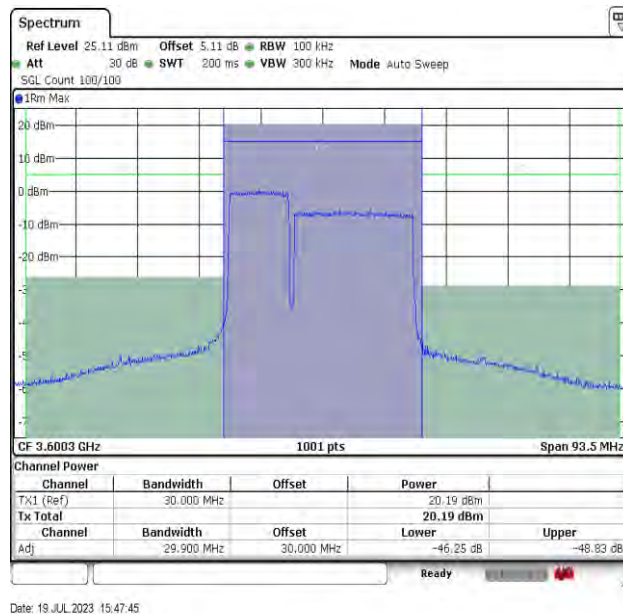
10MHz-20MHz-55896-56040 QPSK-QPSK
