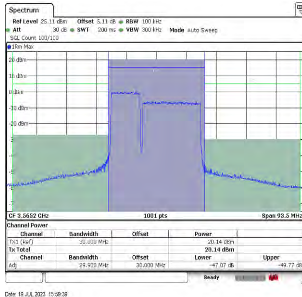
10MHz-20MHz-55295-55439 QPSK-QPSK
