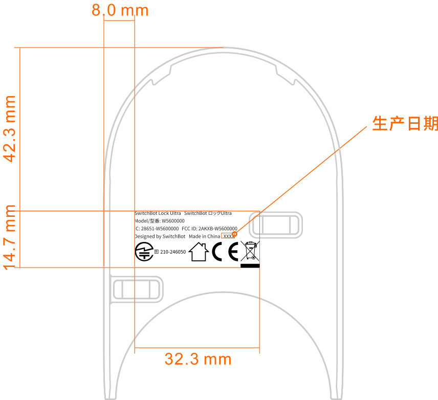
电池盖后视图
