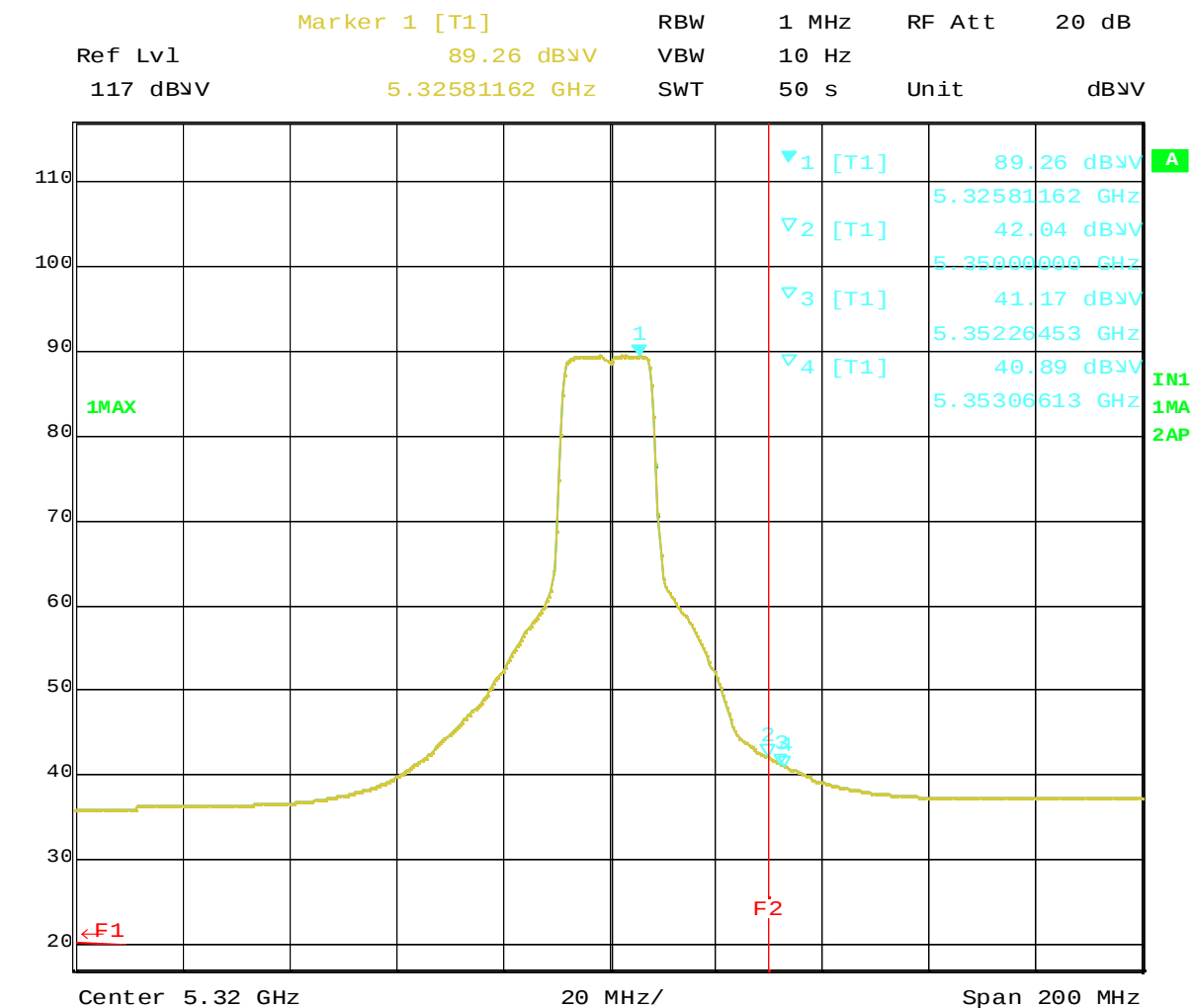
Plot 7-4 5320MHz TX mode (Average). 14" modek
