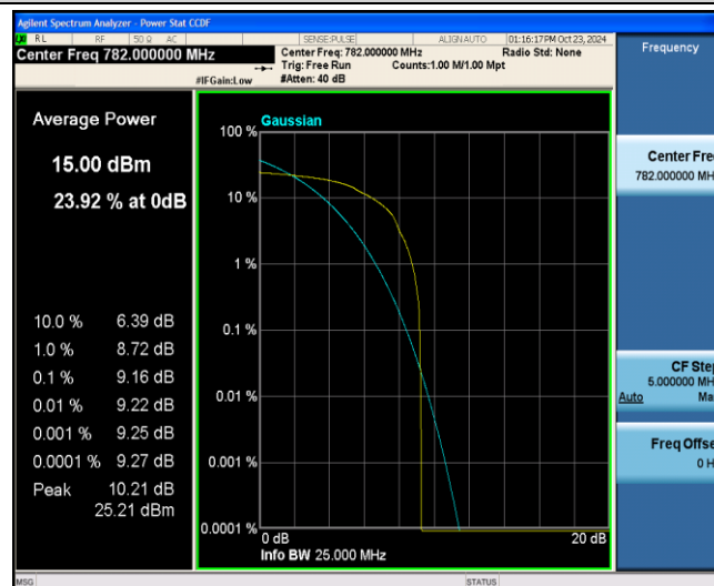
Band13-5MHz-16QAM-23230-1-0-Low-9.16-13-PASS
