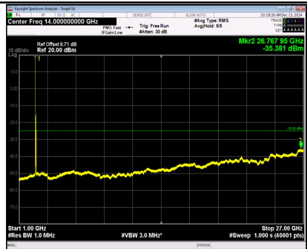
7-7-20MHz-20MHz-QPSK-QPSK-20850-21048-1RB#0-0RB #0-1000~27000MHz-PASS
