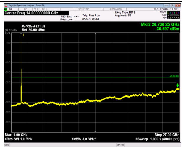
7-7-20MHz-20MHz-QPSK-QPSK-21001-21199-1RB#0-0RB #0-1000~27000MHz-PASS
