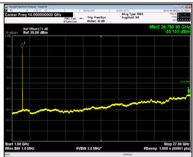
7-7-20MHz-20MHz-QPSK-QPSK-21152-21350-1RB#0-1RB #99-1000~27000MHz-PASS
