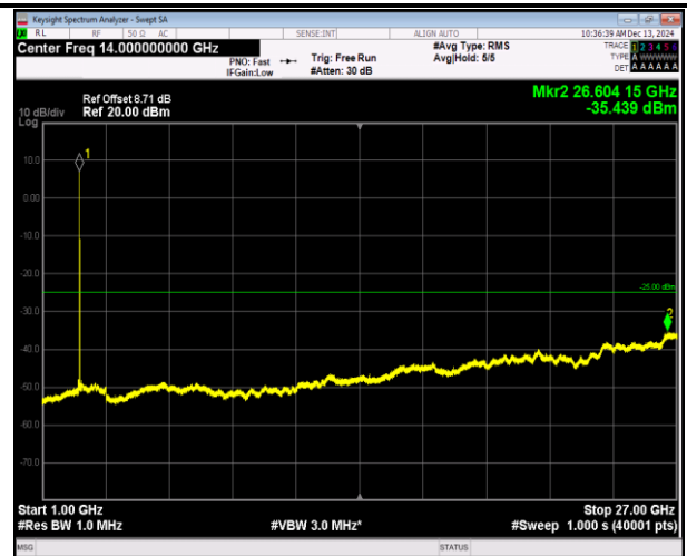
7-7-20MHz-20MHz-QPSK-QPSK-21001-21199-1RB#0-1RB #99-1000~27000MHz-PASS
