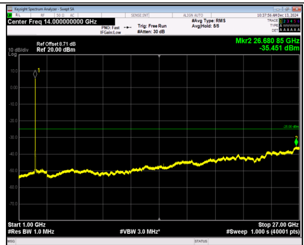
7-7-20MHz-20MHz-QPSK-QPSK-21001-21199-100RB#0-1 00RB#0-1000~27000MHz-PASS
