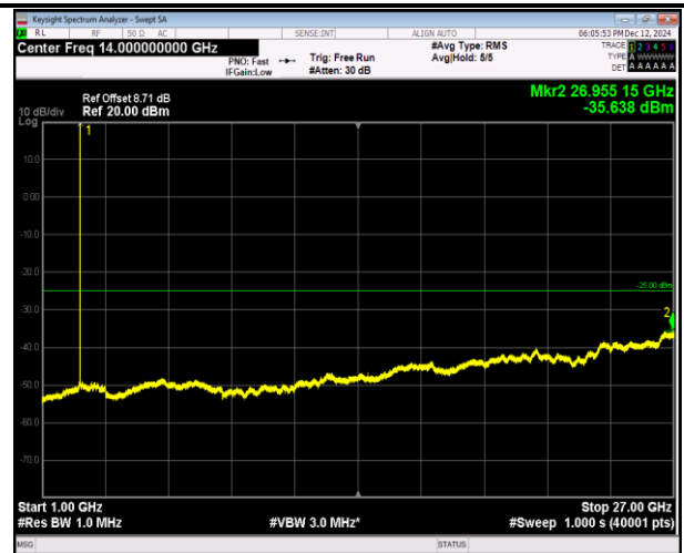
7-7-20MHz-10MHz-QPSK-QPSK-21251-21395-1RB#99-0R B#0-1000~27000MHz-PASS
