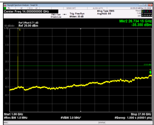
7-7-20MHz-20MHz-QPSK-QPSK-21001-21199-1RB#99-0R B#0-1000~27000MHz-PASS
