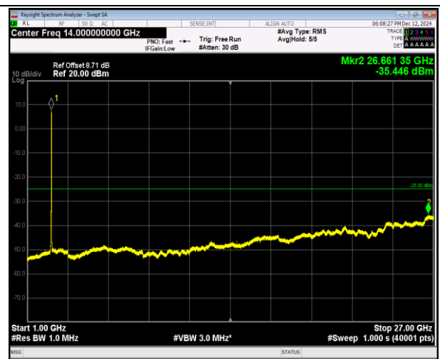
7-7-20MHz-10MHz-QPSK-QPSK-21251-21395-100RB#0-5 0RB#0-1000~27000MHz-PASS
