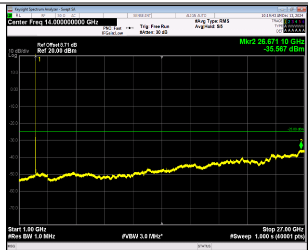
7-7-20MHz-20MHz-QPSK-QPSK-20850-21048-1RB#99-0R B#0-1000~27000MHz-PASS
