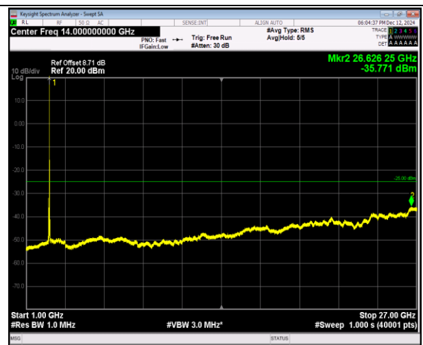
7-7-20MHz-10MHz-QPSK-QPSK-21251-21395-1RB#0-0RB #0-1000~27000MHz-PASS
