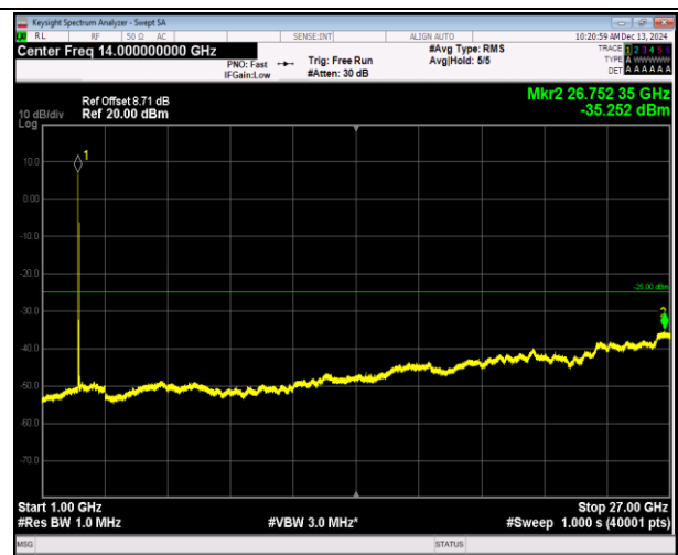
7-7-20MHz-20MHz-QPSK-QPSK-20850-21048-1RB#0-1RB #99-1000~27000MHz-PASS
