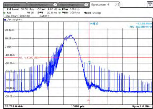
B13_15K_CH23278_QPSK_1RB11_150k
