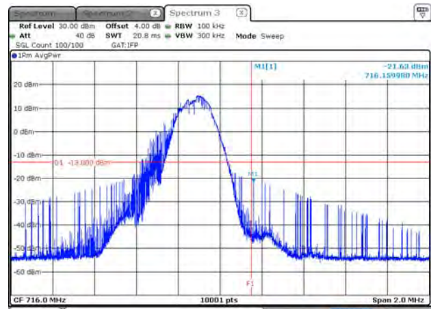
B12_15K_CH23178_QPSK_1RB11_150k
