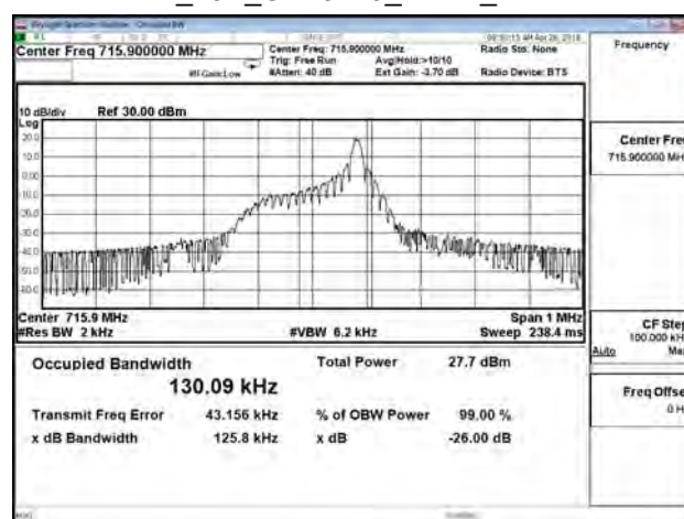
B12_15K_CH23179_BPSK_1RB11
