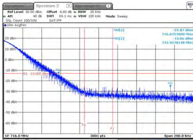
B12_15K_CH23178_BPSK_1RB11_15k
