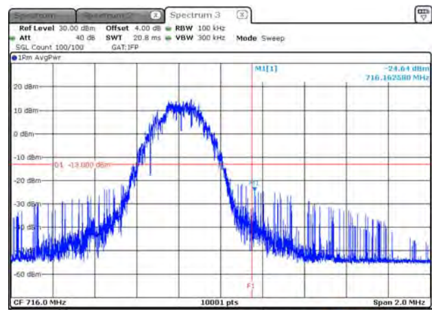
B12_15K_CH23178_QPSK_12RB0_150k
