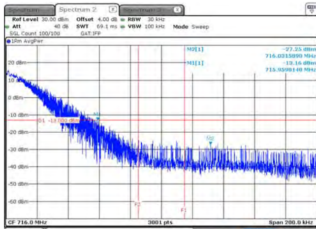
B12_15K_CH23178_QPSK_1RB11_15k
