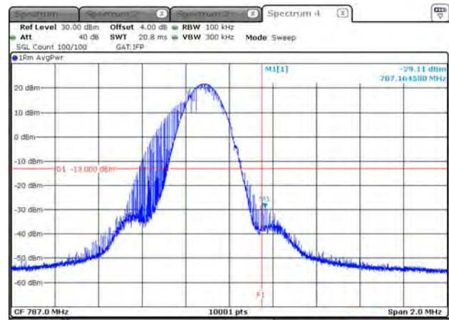
B13_15K_CH23278_BPSK_1RB11_150k
