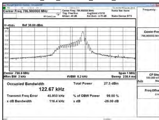
B13_15K_CH23279_QPSK_1RB11
