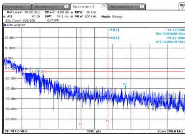
B13_15K_CH23278_QPSK_12RB0_15k
