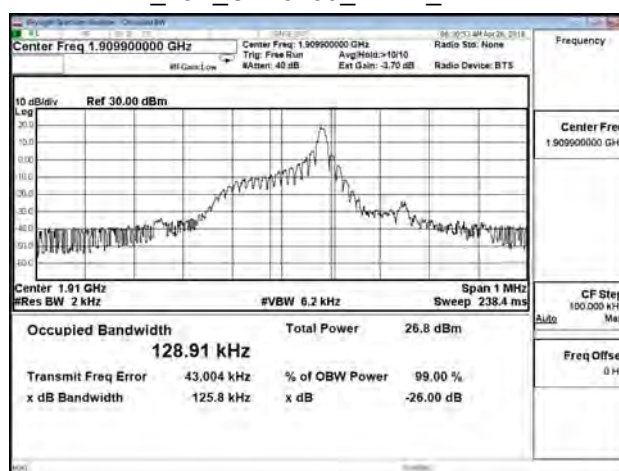
B2_15K_CH19199_BPSK_1RB11
