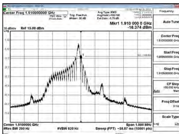
B2_15K_CH19199_QPSK_1RB11
