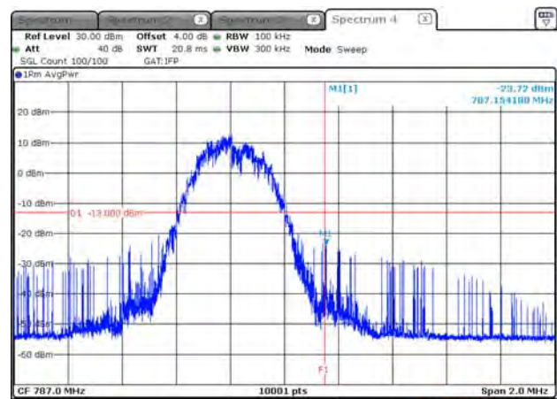
B13_15K_CH23278_QPSK_12RB0_150k
