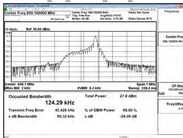
B12_15K_CH23011_BPSK_1RB11
