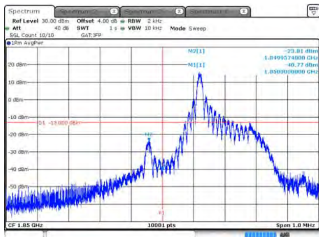
B2_15K_CH18602_BPSK_1RB0
