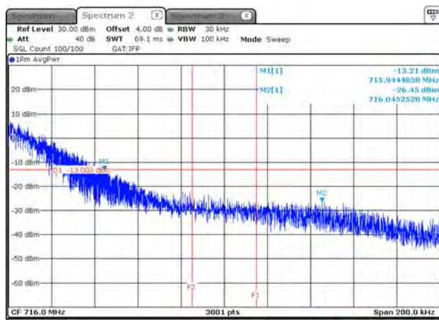
B12_15K_CH23178_QPSK_12RB0_15k
