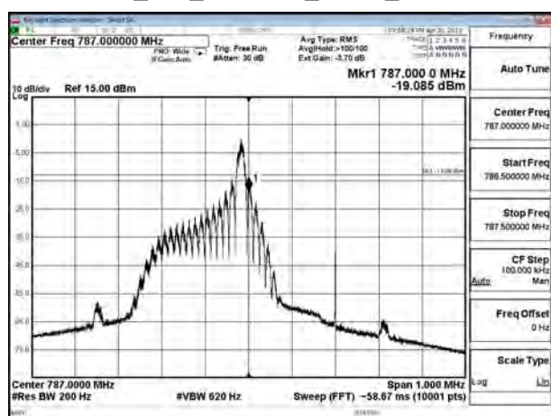
B13_15K_CH23279_QPSK_1RB11
