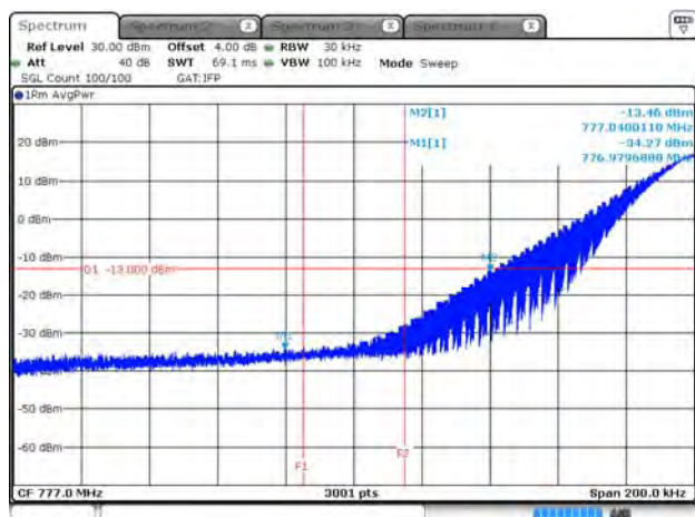
B13_15K_CH23182_BPSK_1RB0_15k
