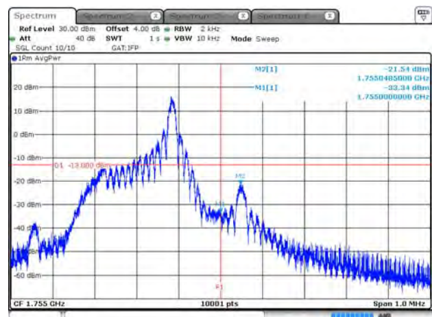
B4_15K_CH20398_BPSK_1RB11
