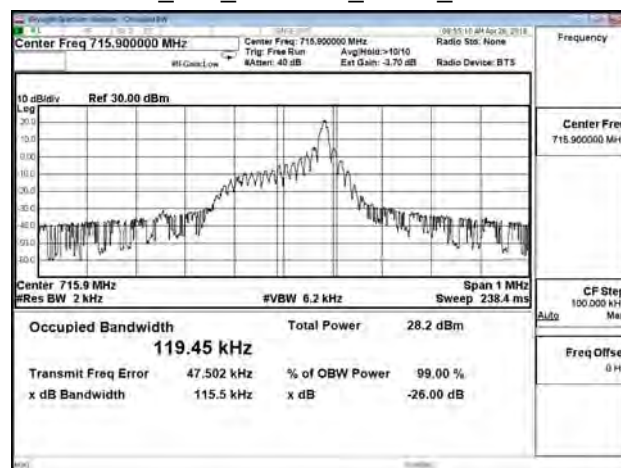
B12_15K_CH23179_QPSK_1RB11
