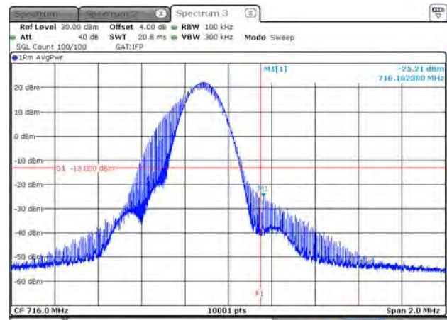
B12_15K_CH23178_BPSK_1RB11_150k
