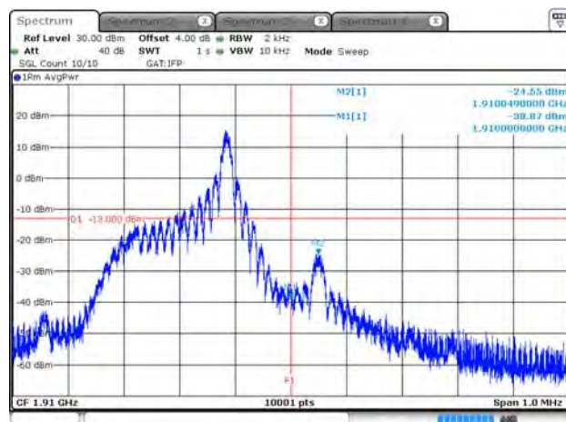
B2_15K_CH19198_BPSK_1RB11
