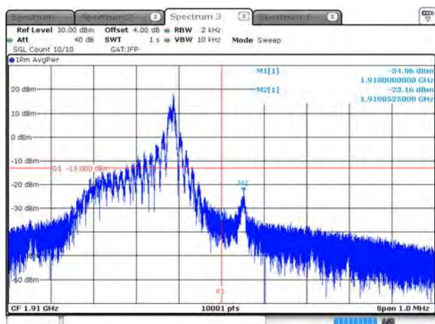
B2_15K_CH19198_QPSK_1RB11
