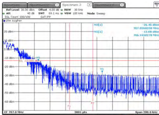
B13_15K_CH23278_QPSK_1RB11_15k
