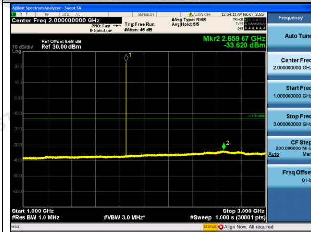
GSM1900-512-0-1000~3000MHz-PASS
