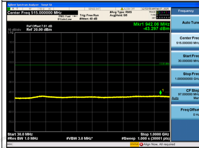
GSM1900-512-0-30~1000MHz-PASS
