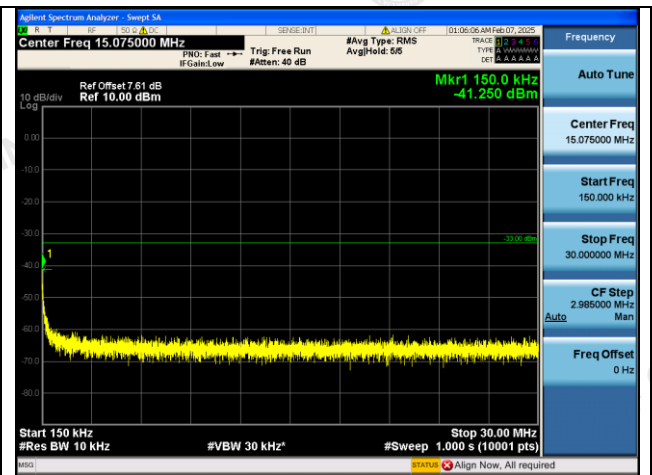
GPRS1900-512-0-0.15~30MHz-PASS
