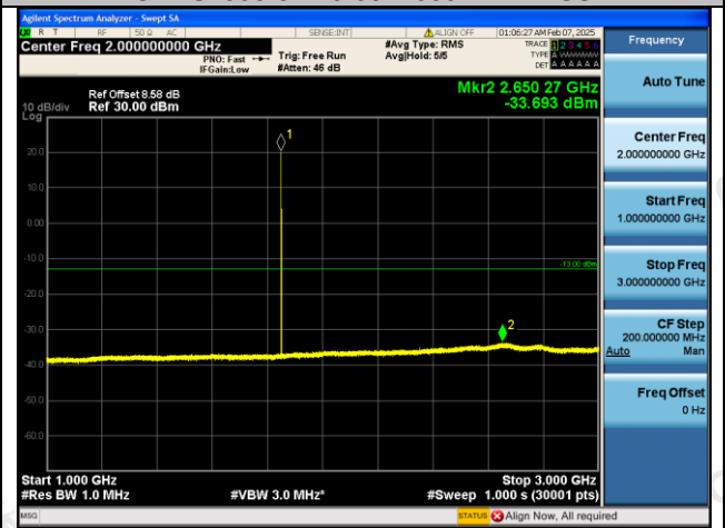
GPRS1900-512-0-1000~3000MHz-PASS
