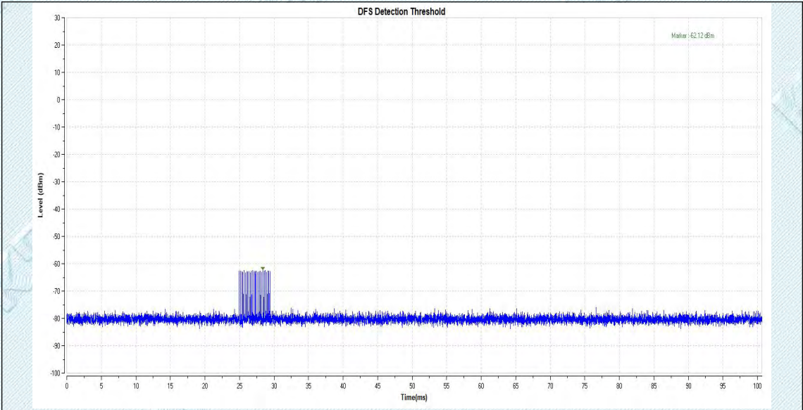
11A_5260_Type3
