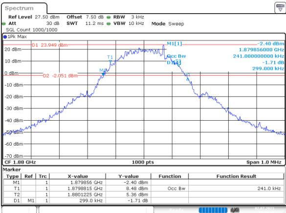
GSM_Middle 0.241MHz
