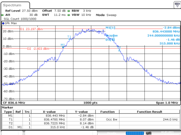
GSM_Middle 0.244MHz
