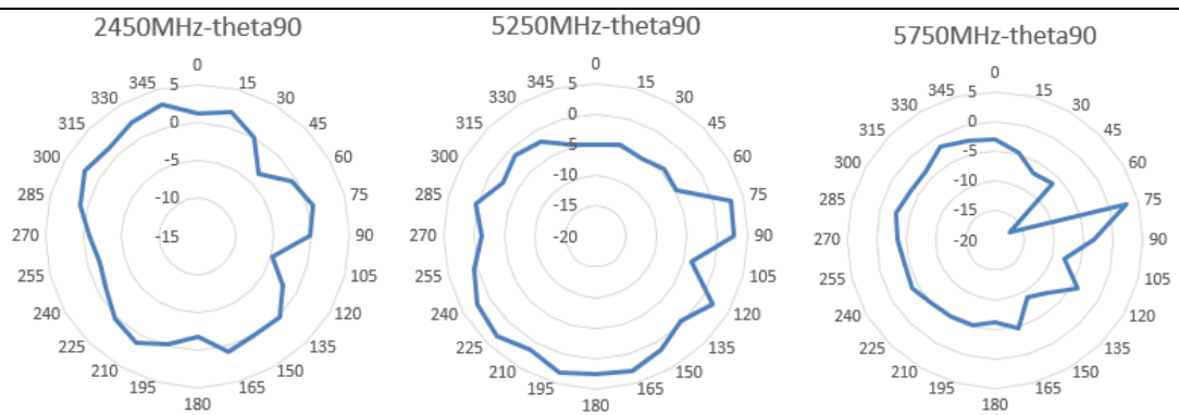
Ant4
