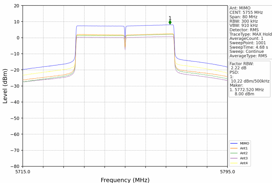
802.11be(EHT40)_LCH_5755MHz_RU484_Left_MIMO_NTNV
