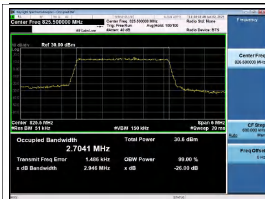
Band26(824-849)-3MHz-QPSK-26805-15RB#0-P ASS
