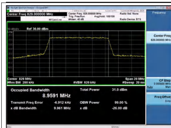
Band26(824-849)-10MHz-QPSK-26840-50RB#0-PASS
