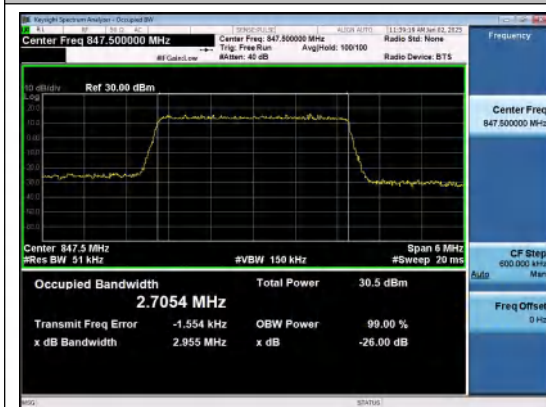
Band26(824-849)-3MHz-QPSK-27025-15RB#0-P ASS
