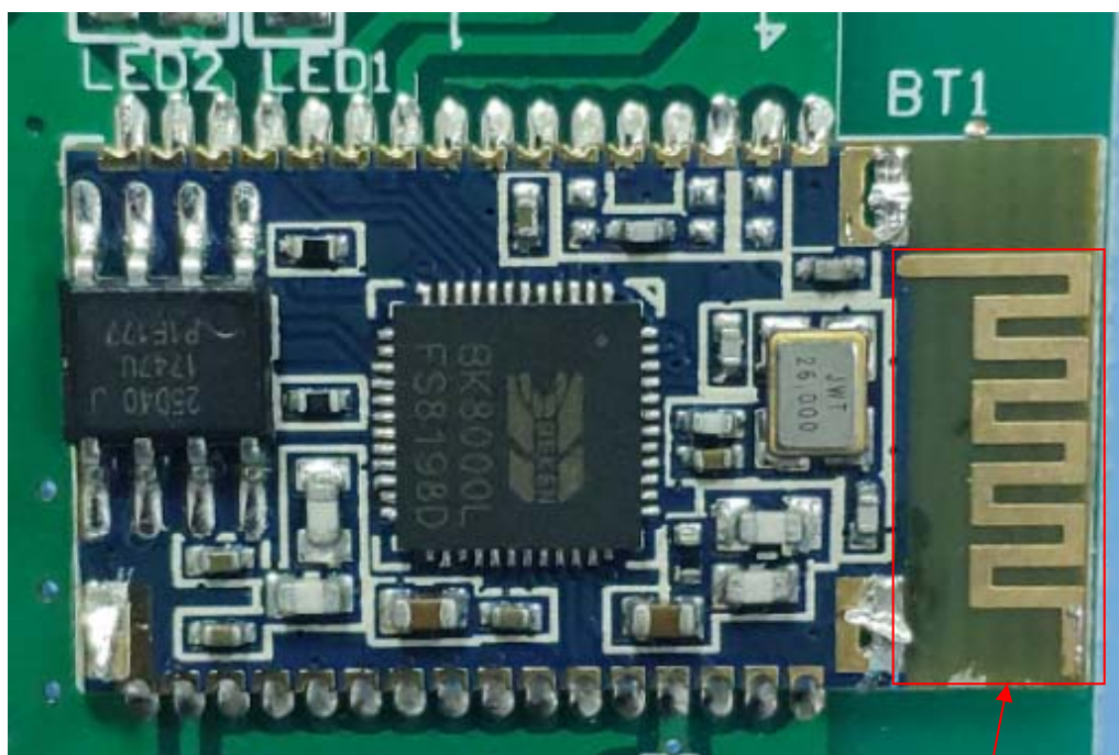
2.4G Antenna
