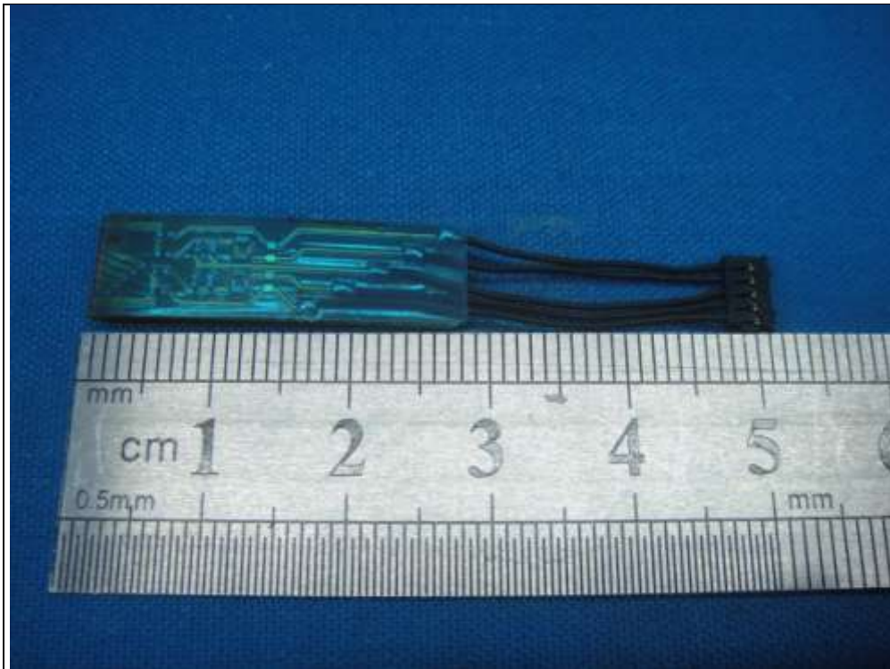
Antenna 1(Brand : SAA / Model : LX8416-12-000-C)
