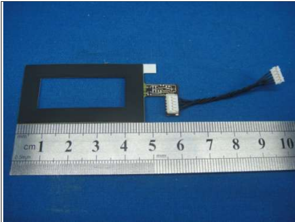
Antenna 5(Brand : SAA / Model : LX7828-12-000-C)
