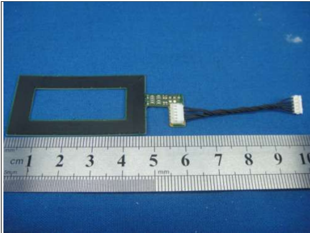
Antenna 2(Brand : Dexerials / Model : ANT-MO41A)
