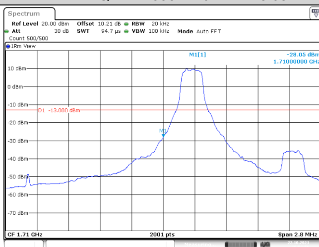
Band4-1.4MHz-QPSK-19957-1-0-Low--28.05-PASS
