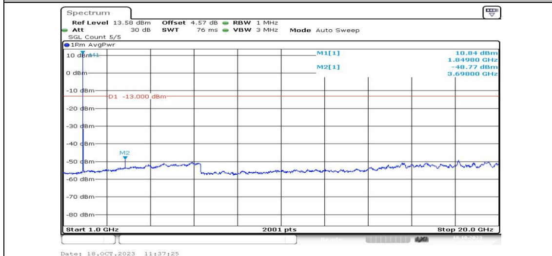
Band2-5MHz-QPSK-18625-1RB#0-Range4:1000~20000MHz-PASS
