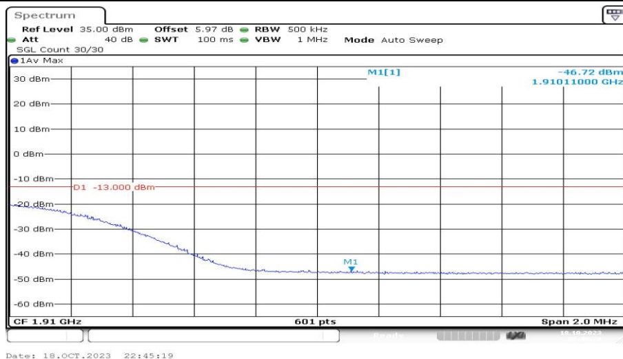
Band2-20MHz-16QAM-19100-1RB#0-PASS
