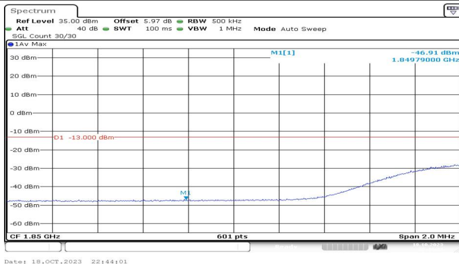
Band2-20MHz-16QAM-18700-1RB#99-PASS
