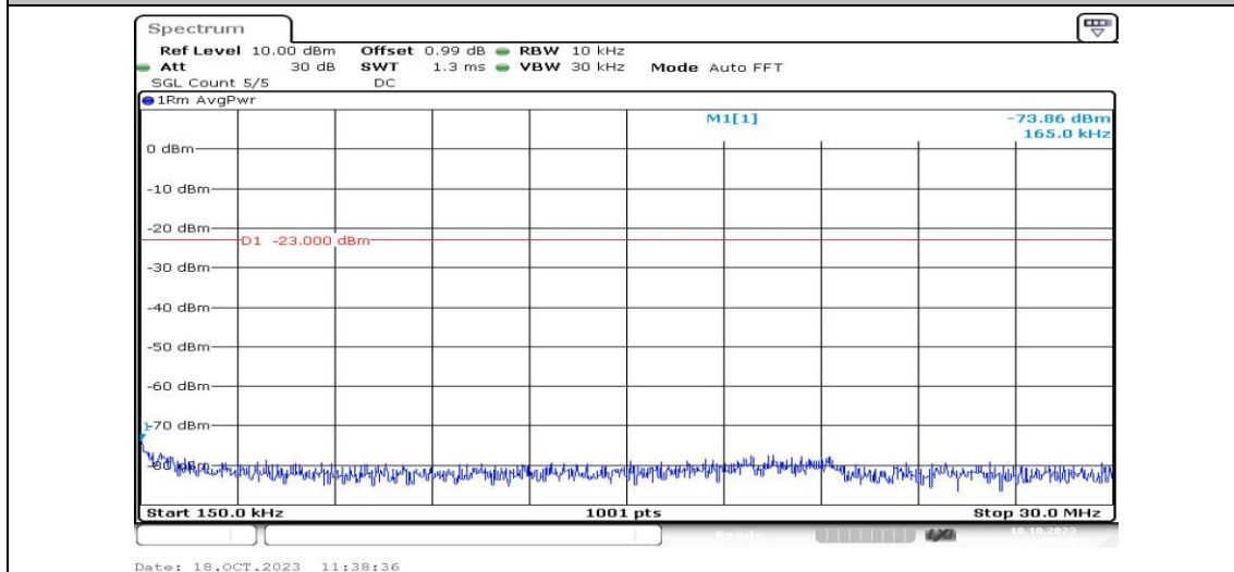
Band2-5MHz-QPSK-18900-1RB#0-Range2:0.15~30MHz-PASS
