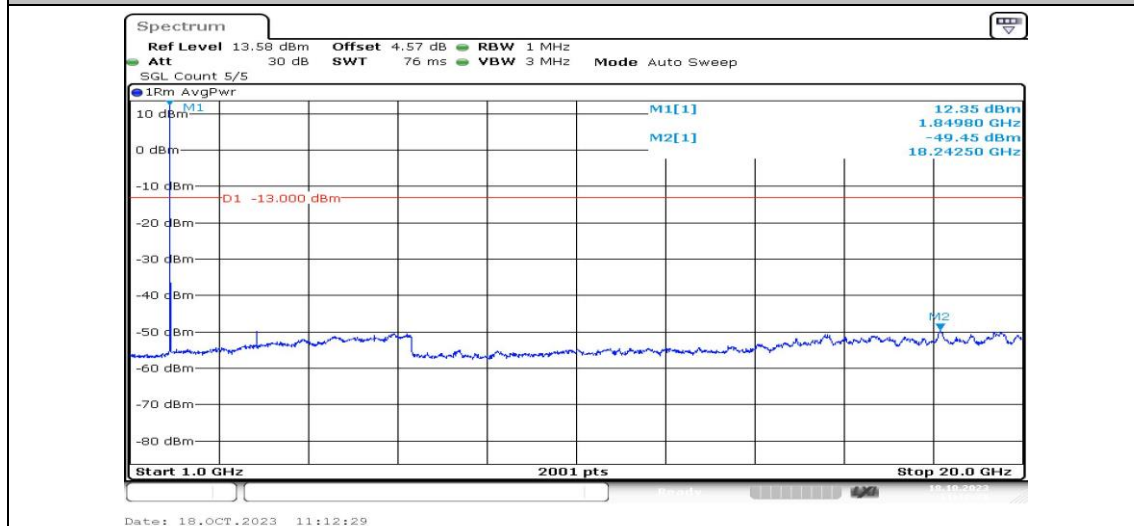
Band2-3MHz-QPSK-18615-1RB#0-Range4:1000~20000MHz-PASS
