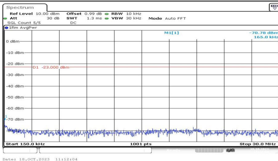
Band2-3MHz-QPSK-18615-1RB#0-Range2:0.15~30MHz-PASS
