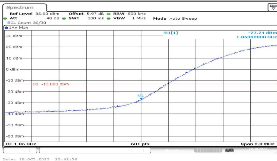
Band2-20MHz-16QAM-18700-1RB#0-PASS
