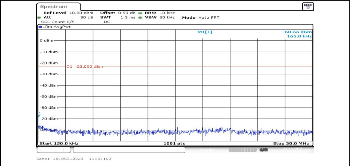
Band2-5MHz-QPSK-18625-1RB#0-Range2:0.15~30MHz-PASS
