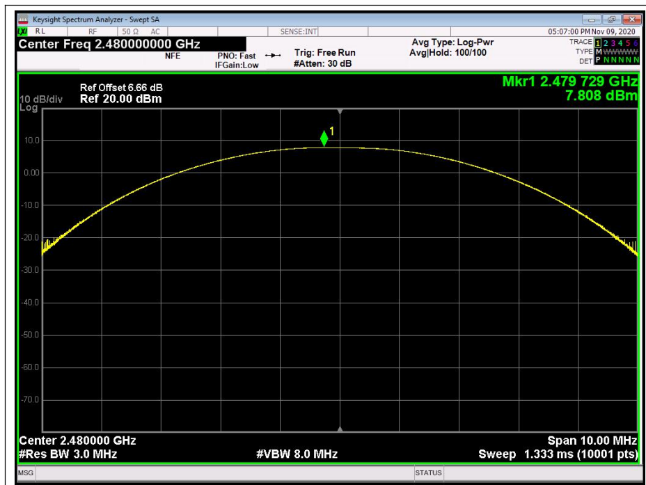
(Channel 39, 2480MHz)
