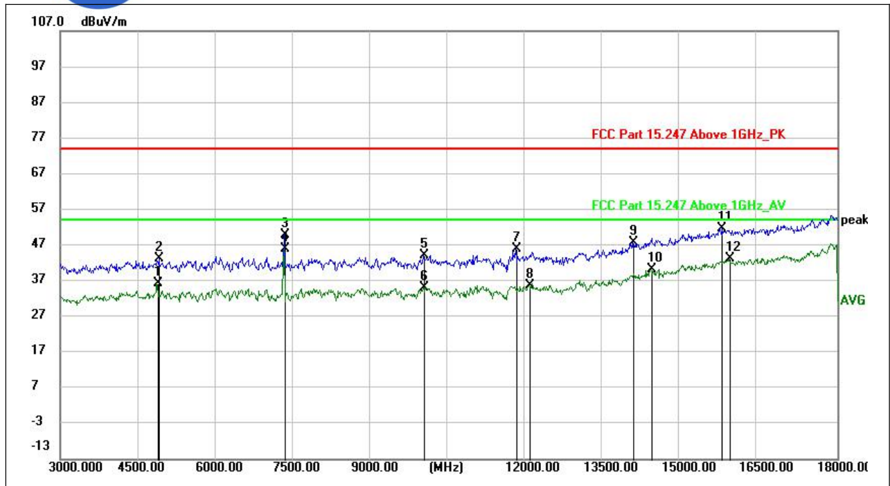
(LE 1M PHY_2442MHz, Antenna Horizontal, 3GHz to 18GHz)
