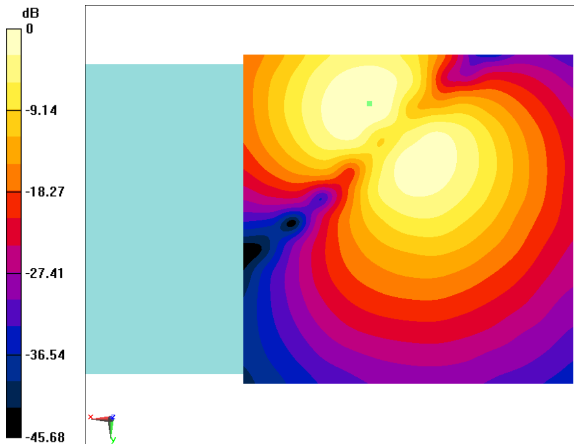
Fig B.8 T-Coil WCDMA 1700
